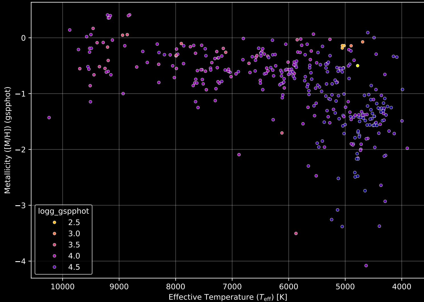
Gaia Cluster: [NGC_6728] Stellar Population Parameters (n= 357)
