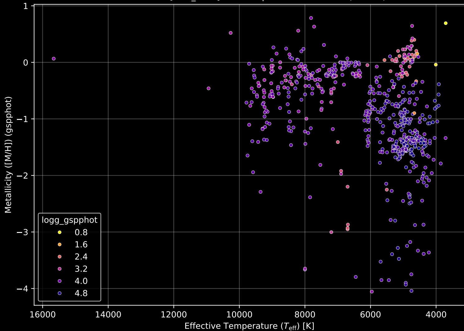
Gaia Cluster: [NGC_6735] Stellar Population Parameters (n= 608)
