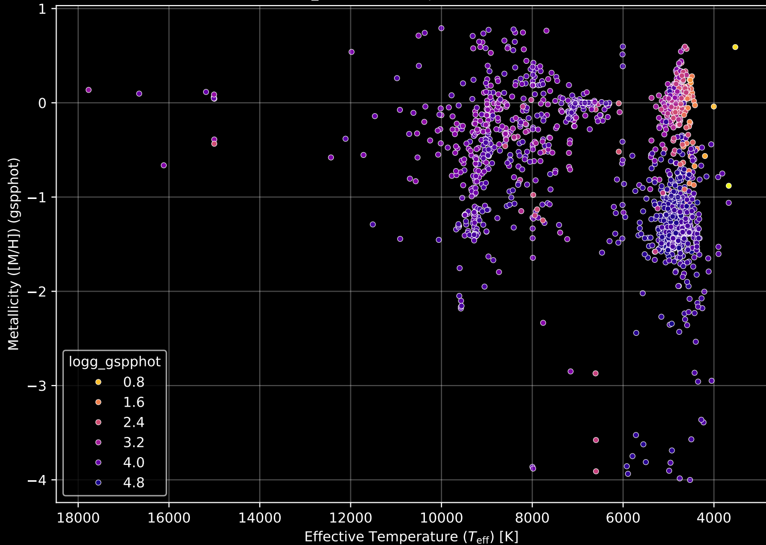
Gaia Cluster: [NGC_6755] Stellar Population Parameters (n= 1379)
