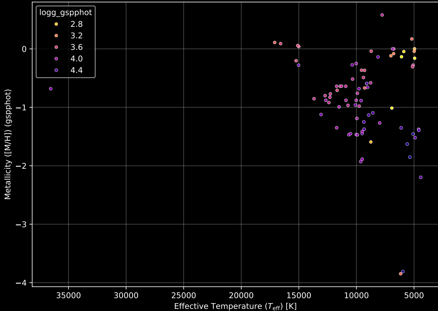
Gaia Cluster: [NGC_7067] Stellar Population Parameters (n= 81)
