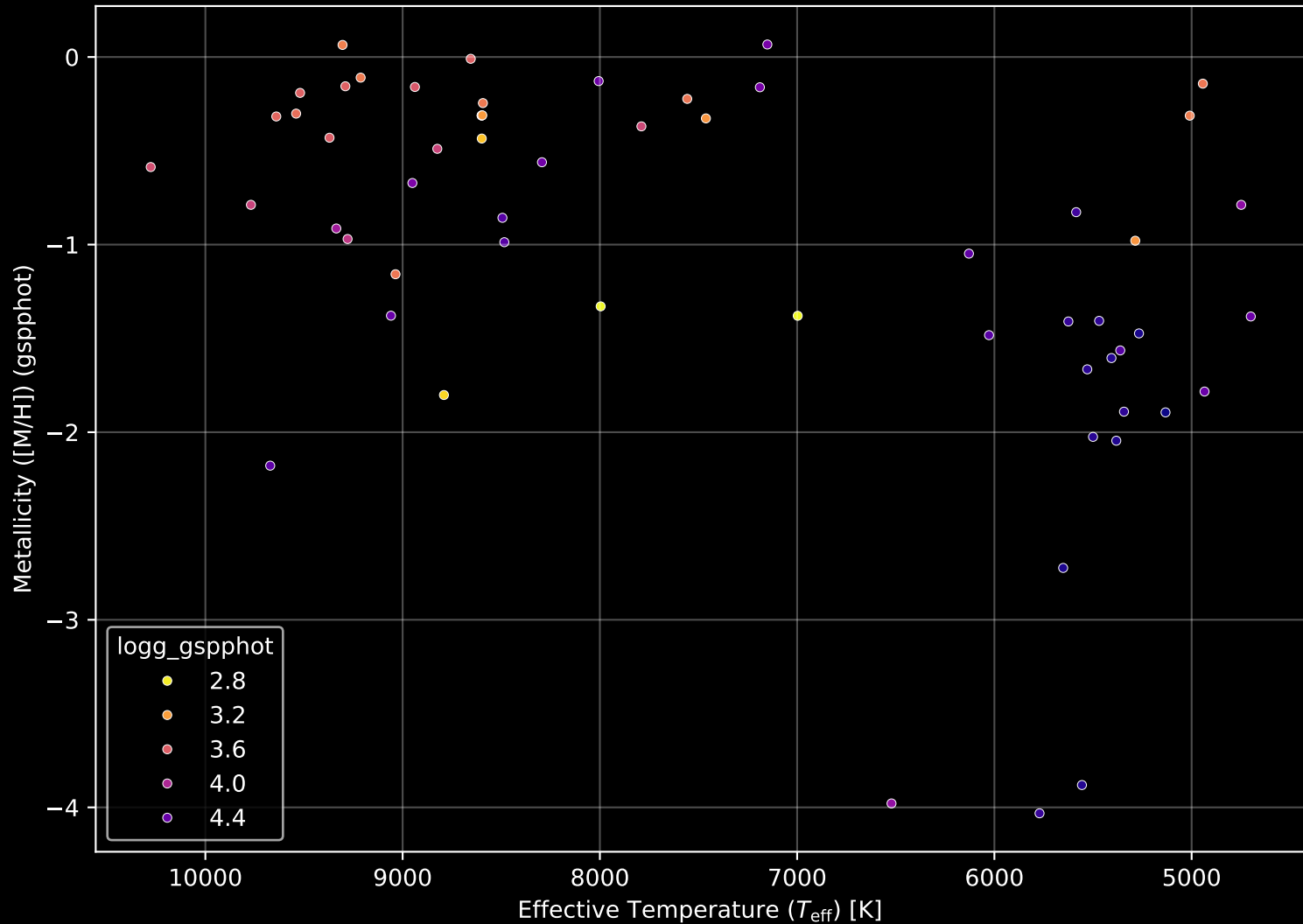
Gaia Cluster: [NGC_7226] Stellar Population Parameters (n= 58)
