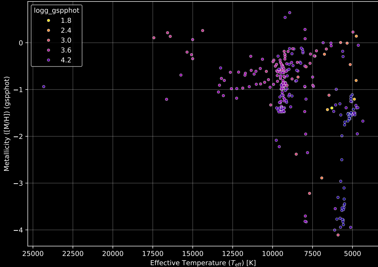
Gaia Cluster: [NGC_7235] Stellar Population Parameters (n= 262)
