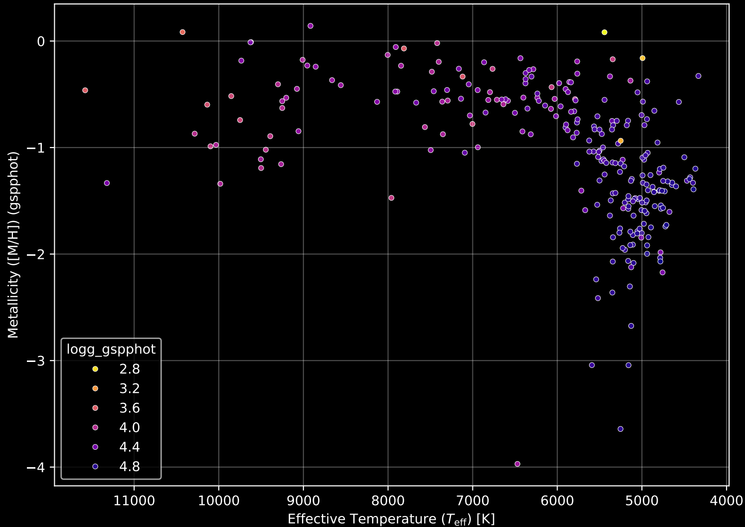
Gaia Cluster: [NGC_7296] Stellar Population Parameters (n= 257)
