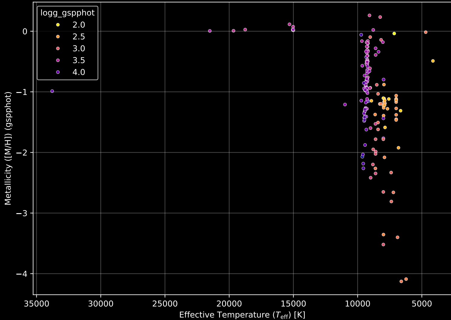
Gaia Cluster: [NGC_7419] Stellar Population Parameters (n= 180)
