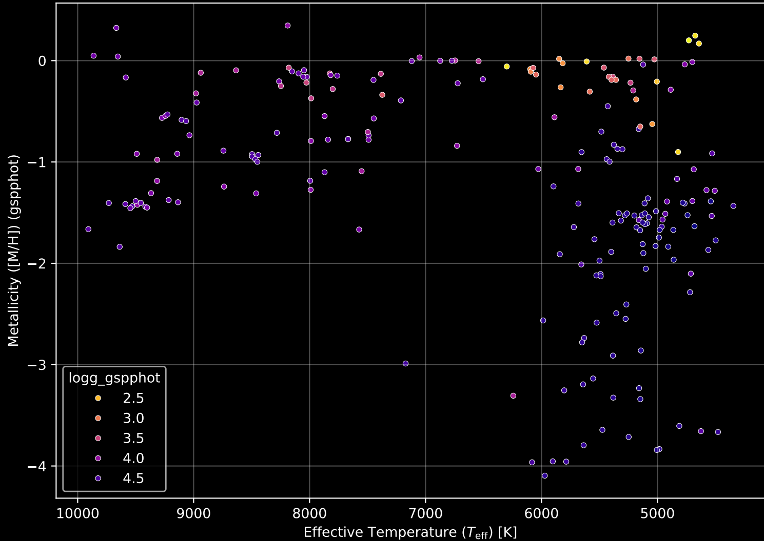
Gaia Cluster: [NGC_7423] Stellar Population Parameters (n= 215)
