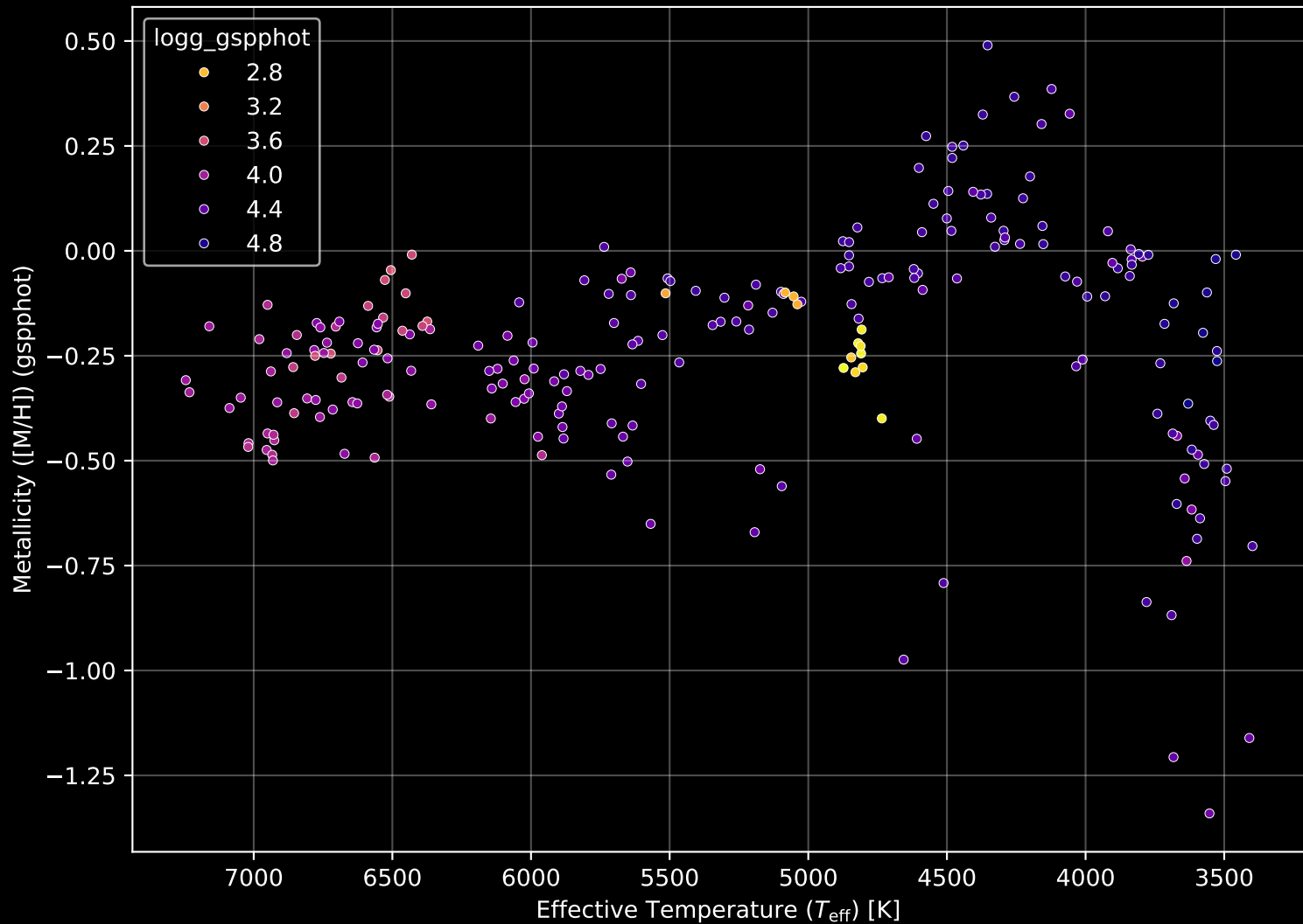
Gaia Cluster: [NGC_752] Stellar Population Parameters (n= 232)
