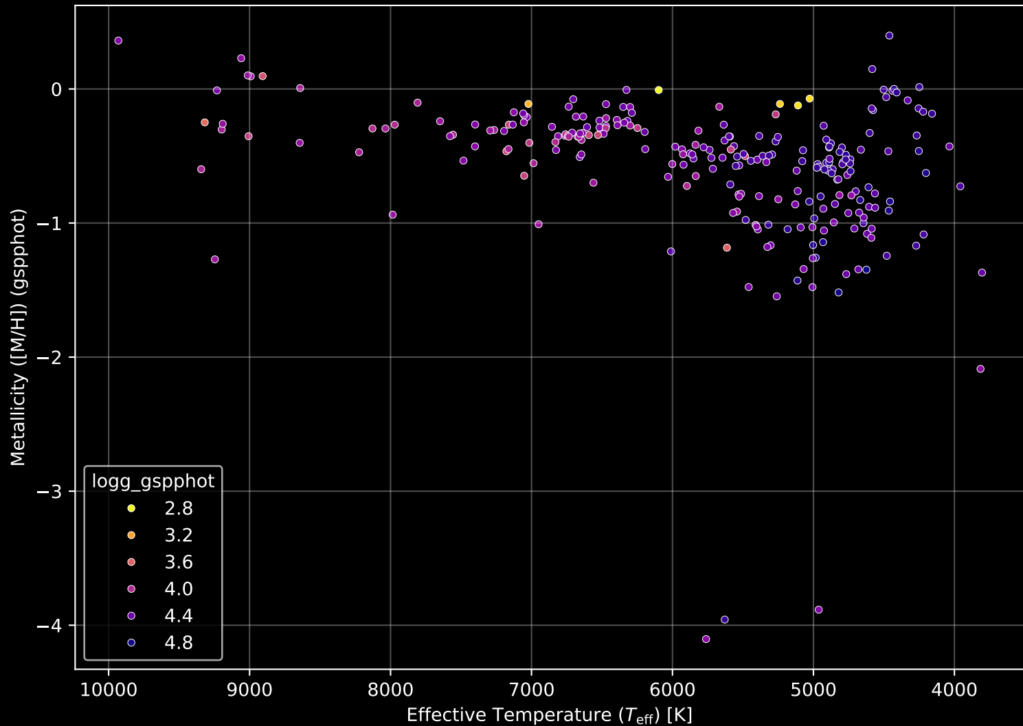
Gaia Cluster: [NGC_886] Stellar Population Parameters (n= 251)
