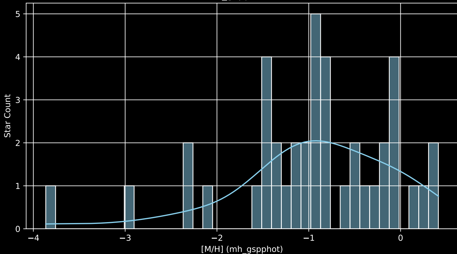
Gaia Cluster: [Pfleiderer_3 [M/H] (mh_gspphot) (n= 41)
