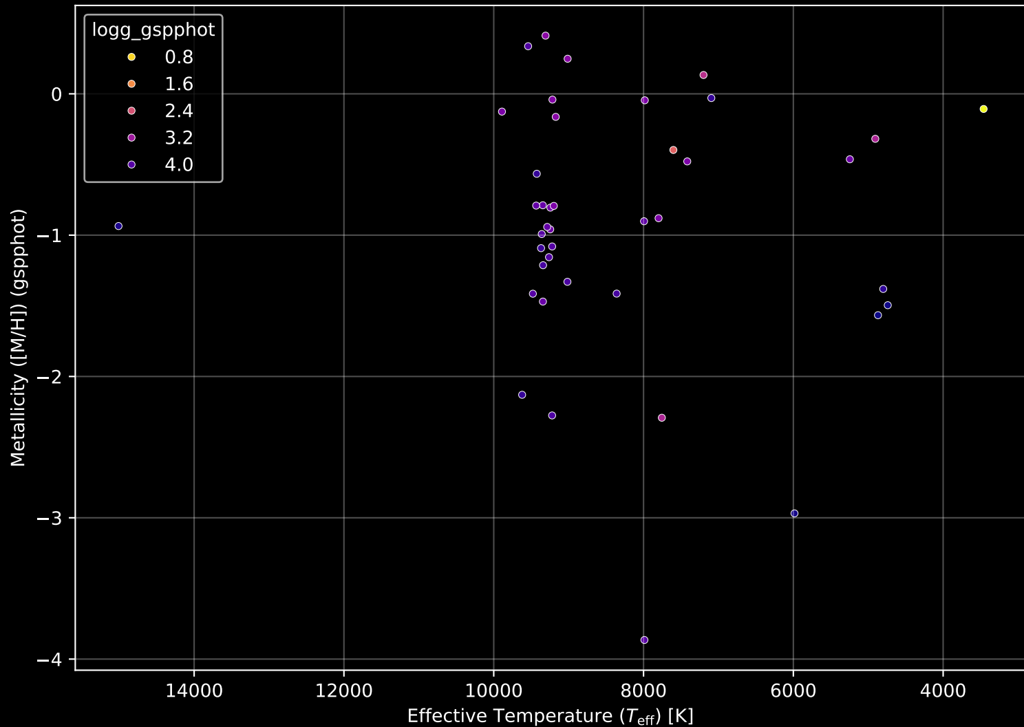
Gaia Cluster: [Pfleiderer_3] Stellar Population Parameters (n= 41)
