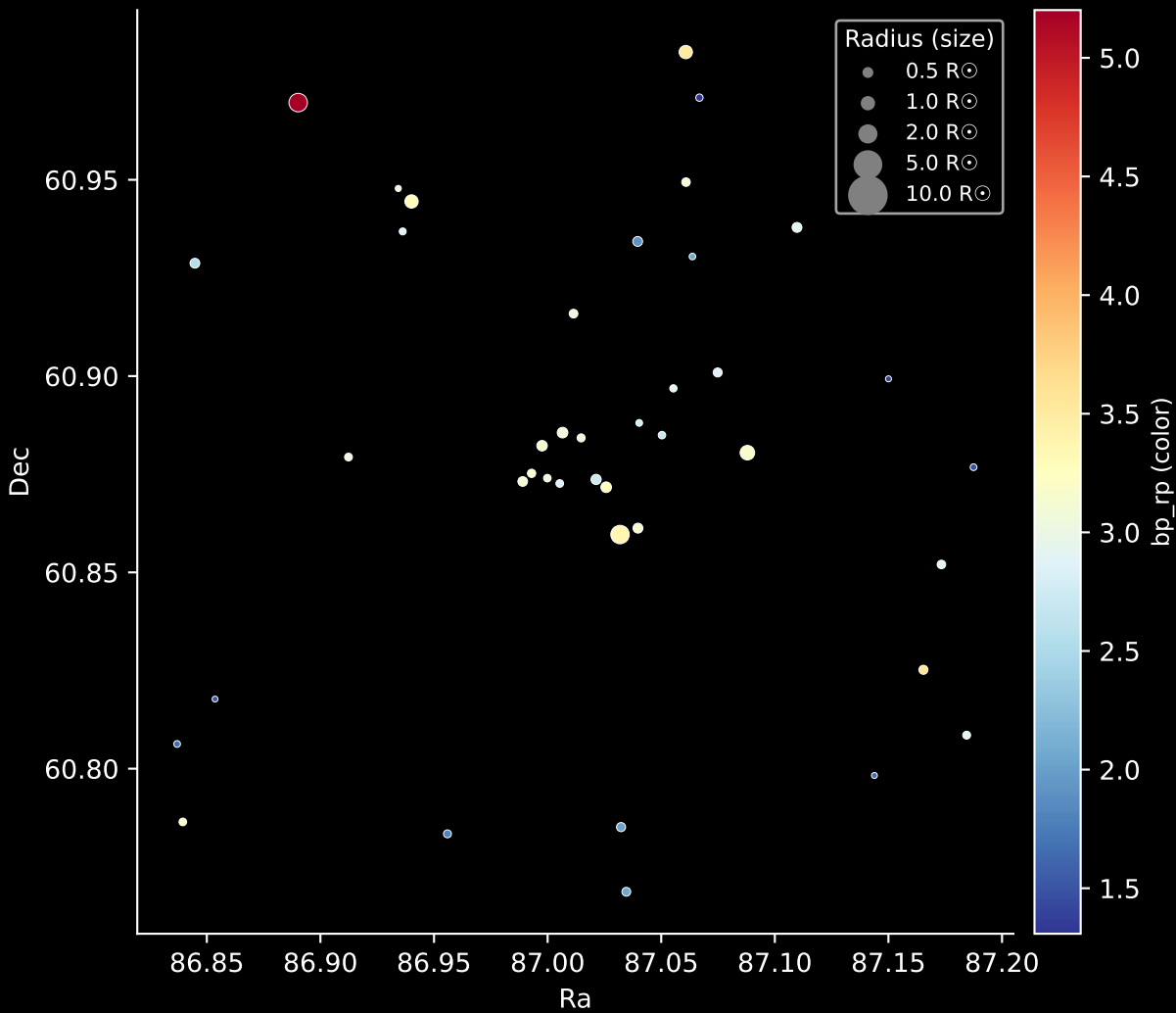
Gaia Cluster: [Pfleiderer_3] Stars: 41
