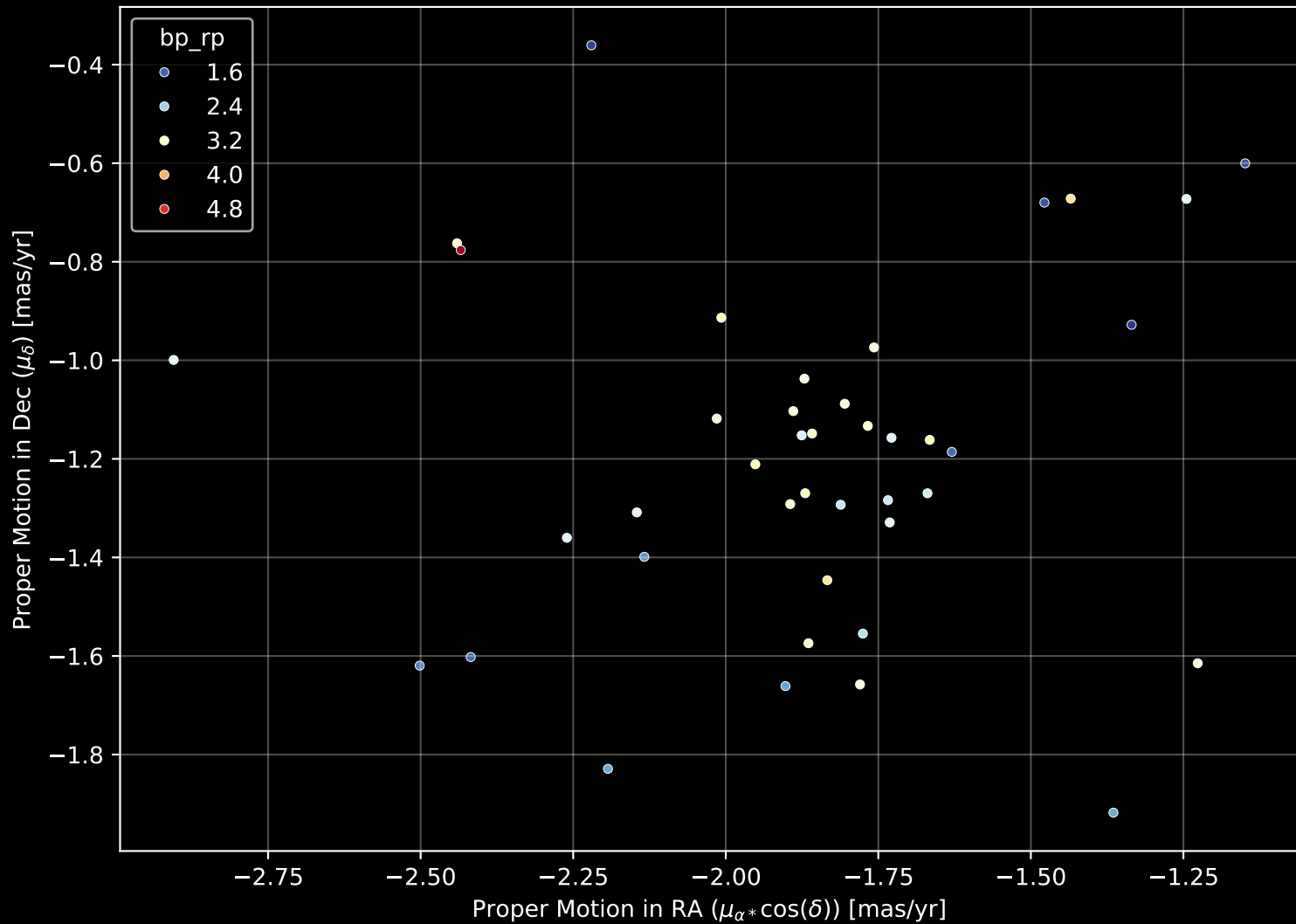
Gaia Cluster: [Pfleiderer_3] Proper Motion Diagram (n= 41)
