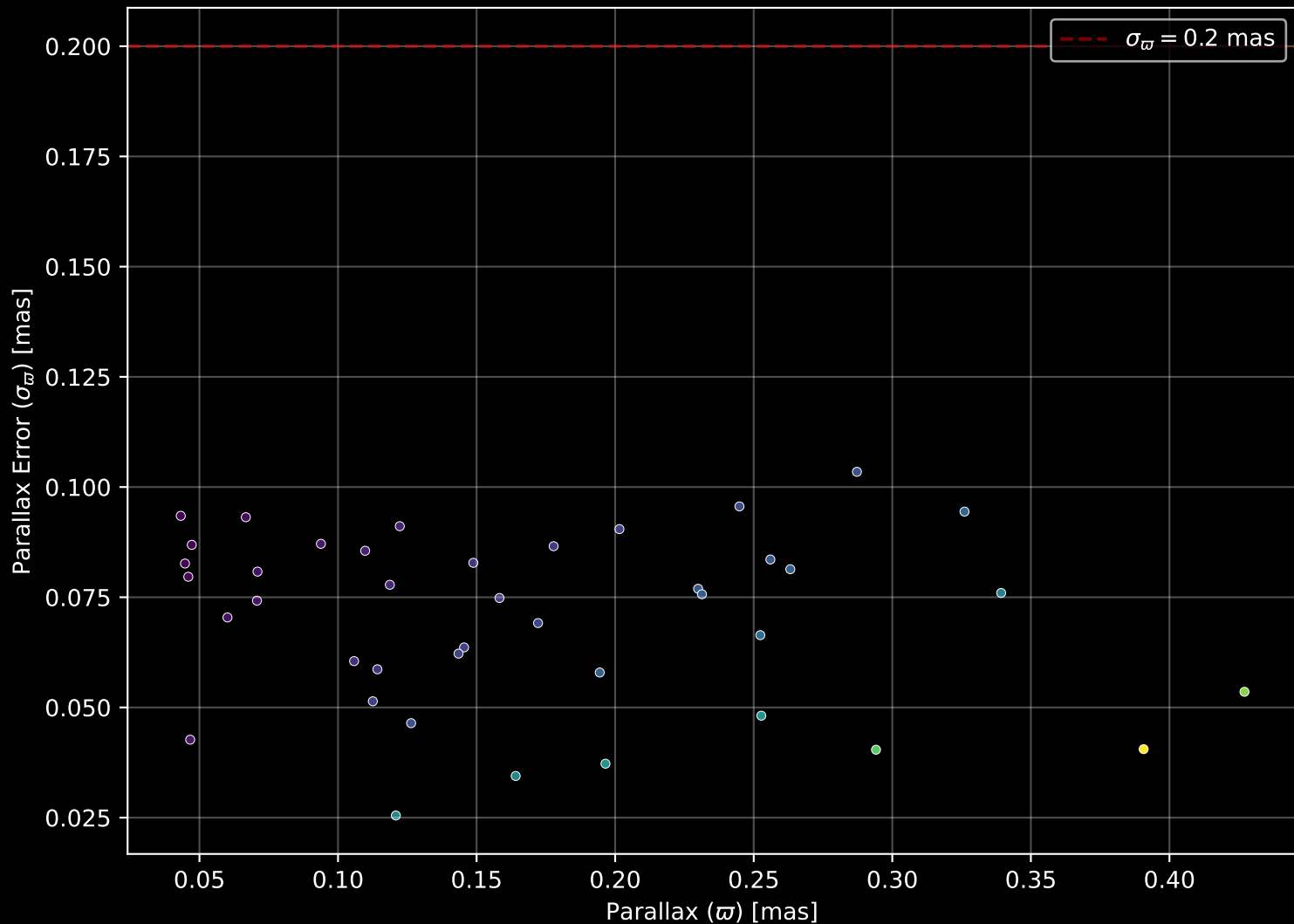
Gaia Cluster: [Pfleiderer_3] Parallax Quality (n= 41)
