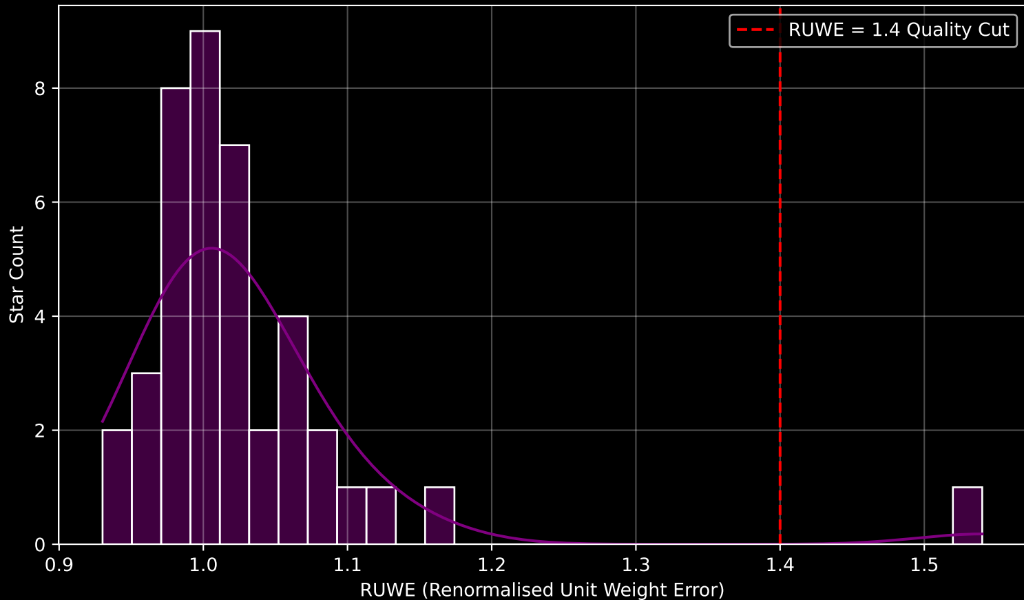
Gaia Cluster: [Pfleiderer_3] RUWE Distribution (n= 41)
