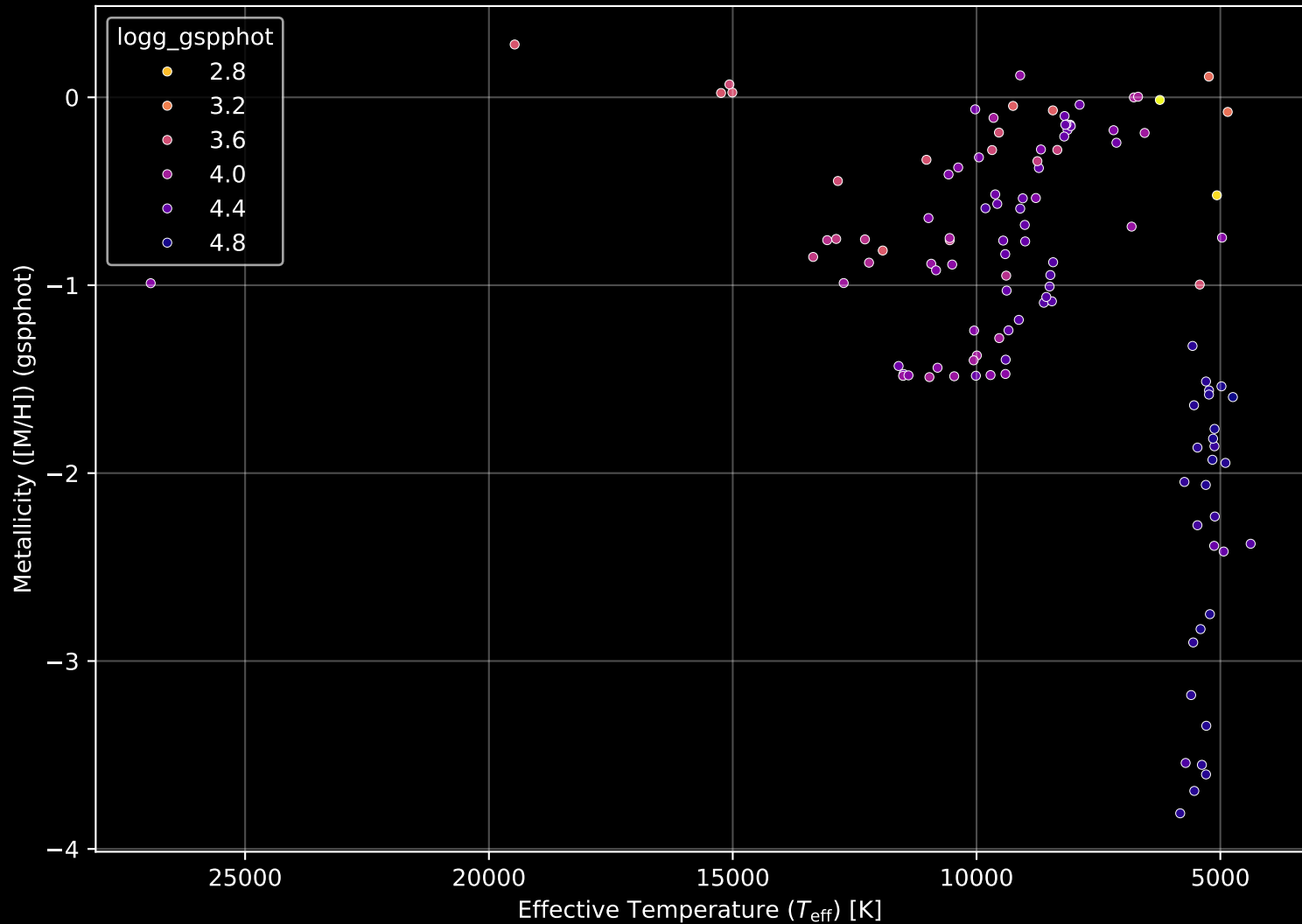
Gaia Cluster: [Pismis_1] Stellar Population Parameters (n= 120)
