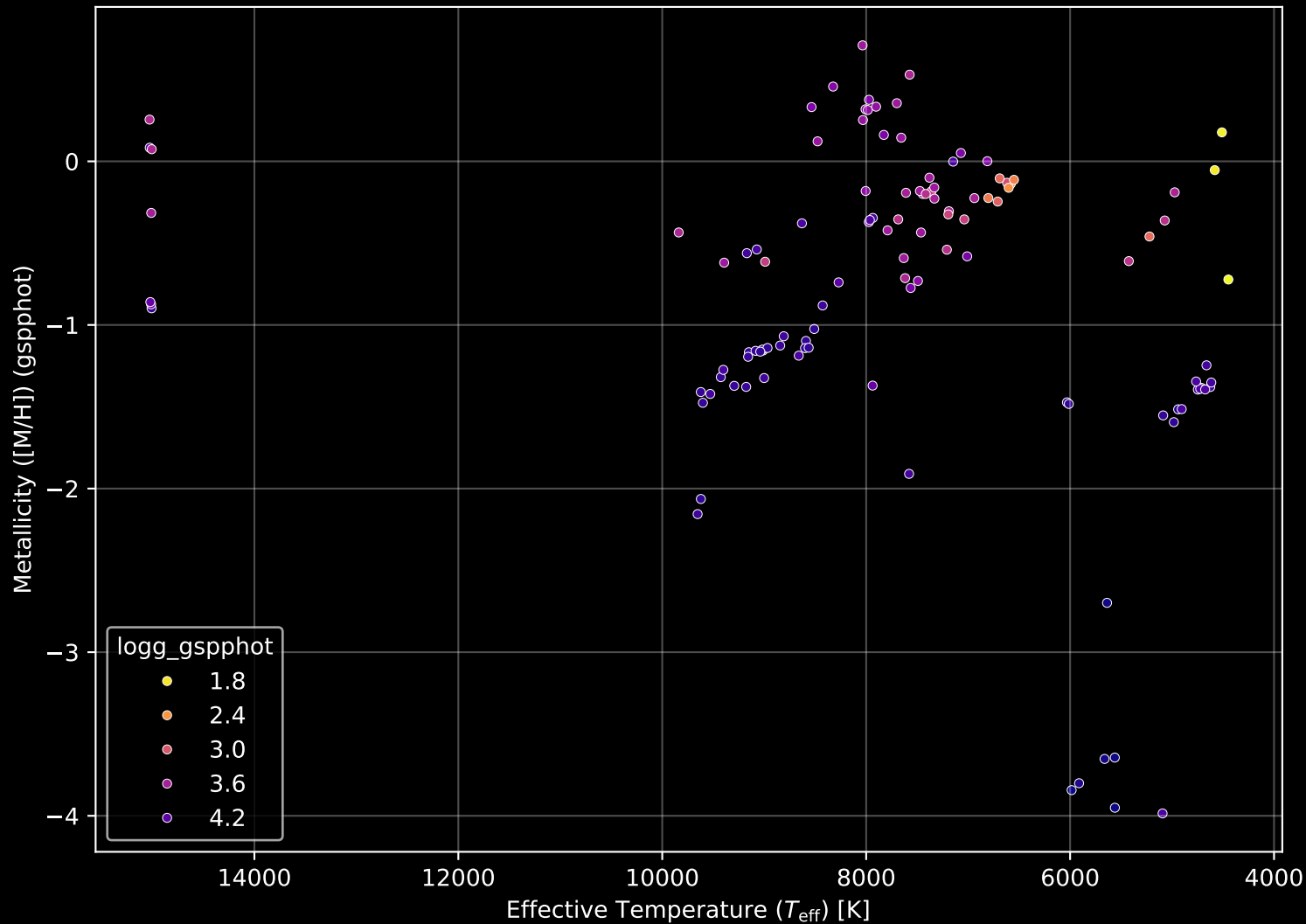
Gaia Cluster: [Pismis_2] Stellar Population Parameters (n= 118)
