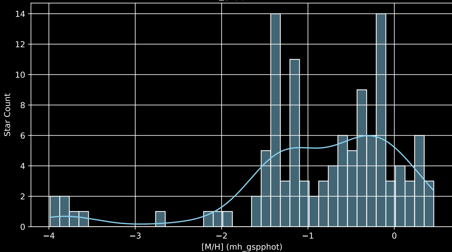
Gaia Cluster: [Pismis_2 [M/H] (mh_gspphot) (n= 116)
