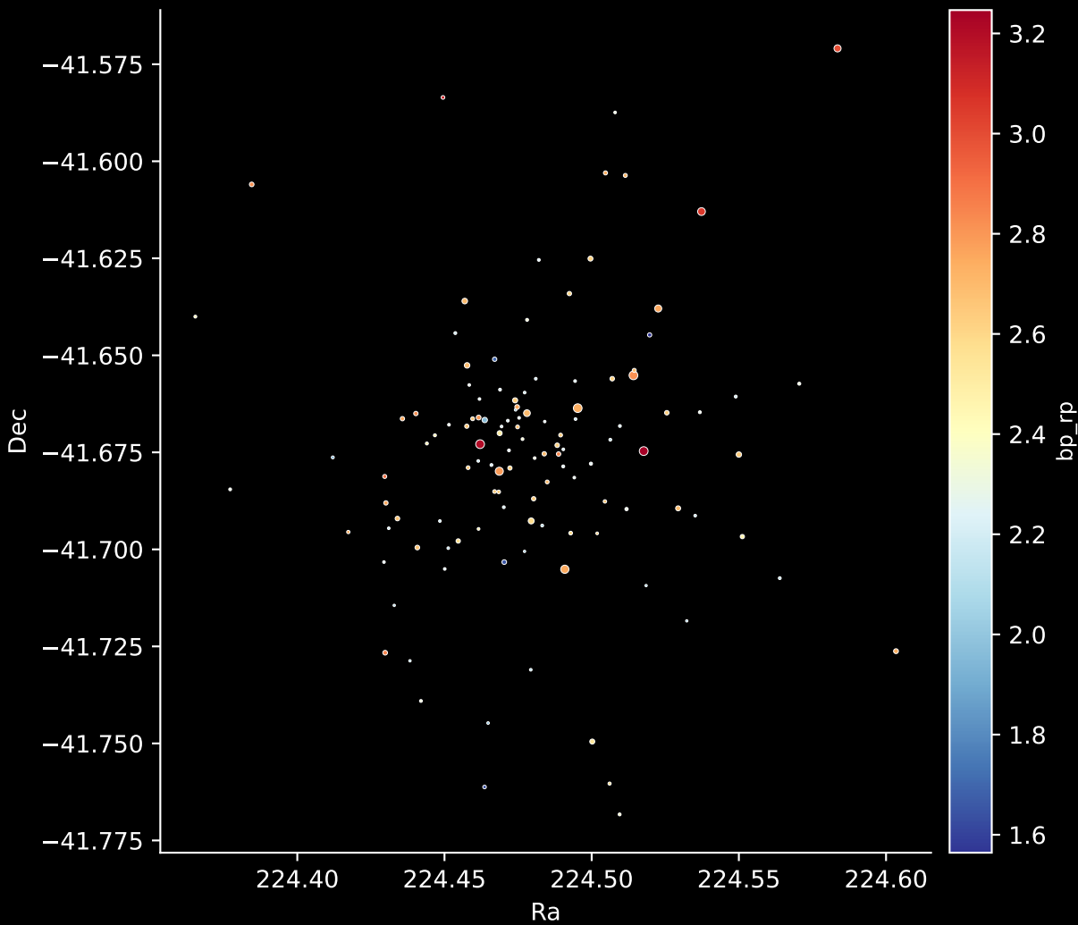
Gaia Cluster: [Pismis_2] Stars: 118
