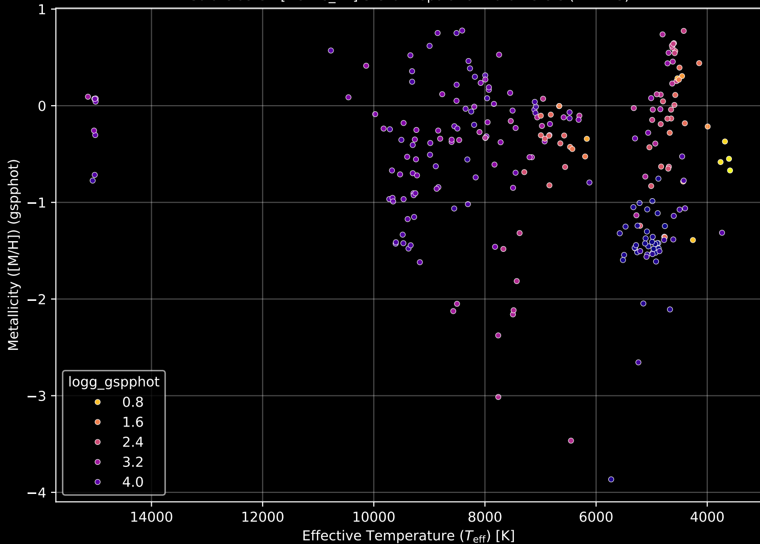
Gaia Cluster: [Pismis_22] Stellar Population Parameters (n= 243)
