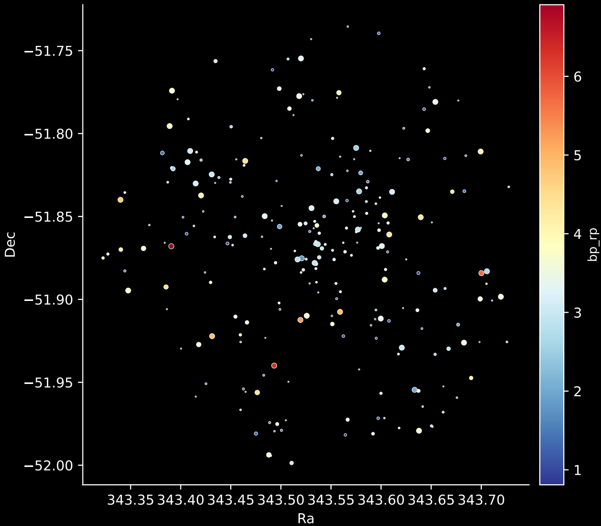
Gaia Cluster: [Pismis_22] Stars: 243
