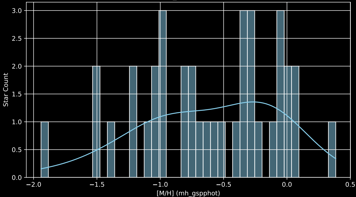
Gaia Cluster: [Pismis_Moreno_1 [M/H] (mh_gspphot) (n= 37)
