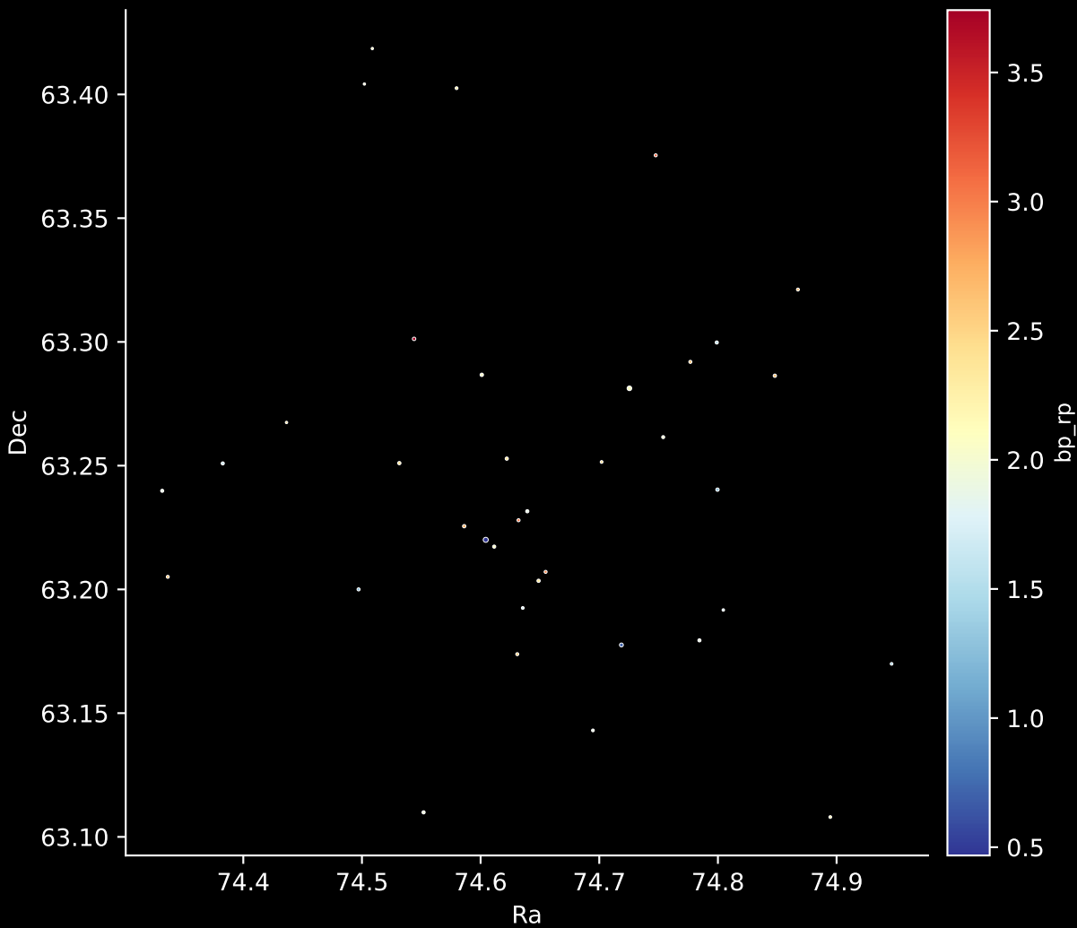
Gaia Cluster: [Pismis_Moreno_1] Stars: 37
