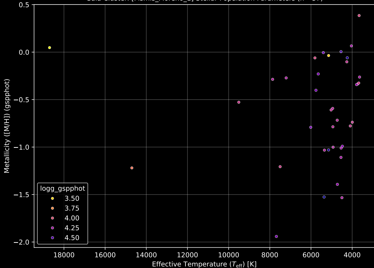
Gaia Cluster: [Pismis_Moreno_1] Stellar Population Parameters (n= 37)
