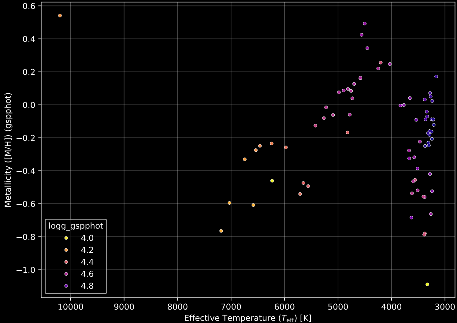
Gaia Cluster: [Platais_3] Stellar Population Parameters (n= 75)
