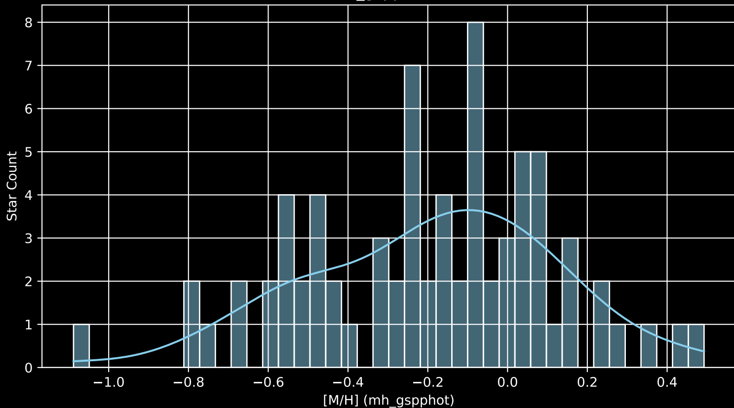
Gaia Cluster: [Platais_3 [M/H] (mh_gspphot) (n= 74)
