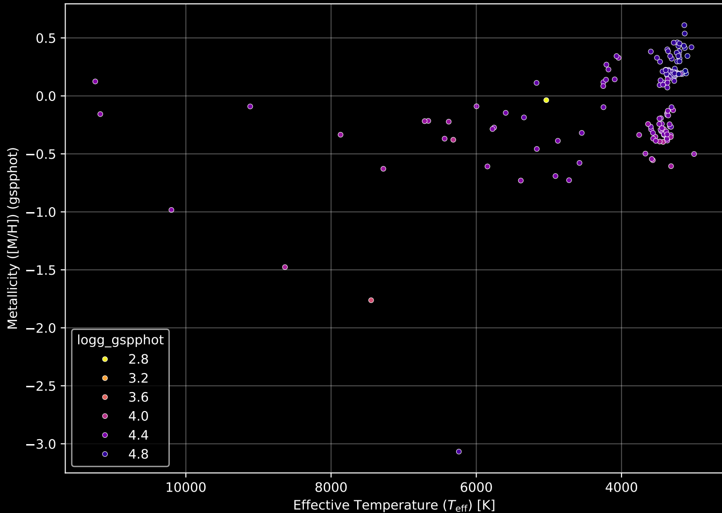
Gaia Cluster: [Platais_8] Stellar Population Parameters (n= 160)
