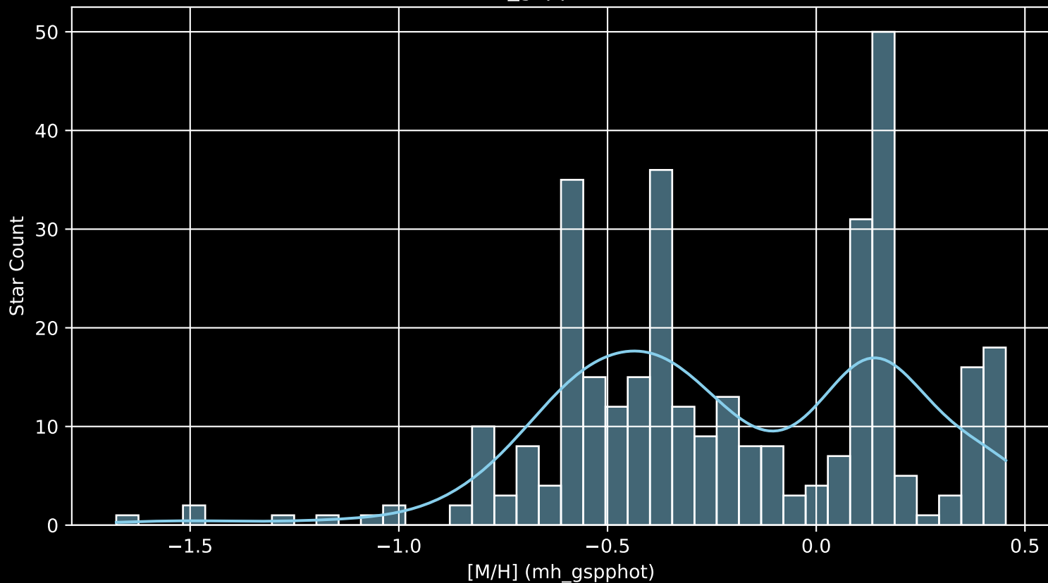
Gaia Cluster: [Pozzo_1 [M/H] (mh_gspphot) (n= 336)
