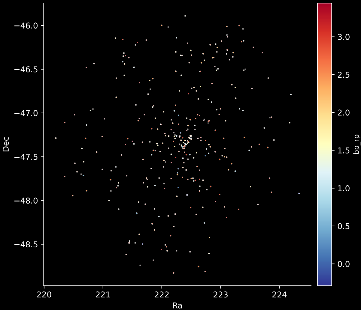
Gaia Cluster: [Pozzo_1] Stars: 338
