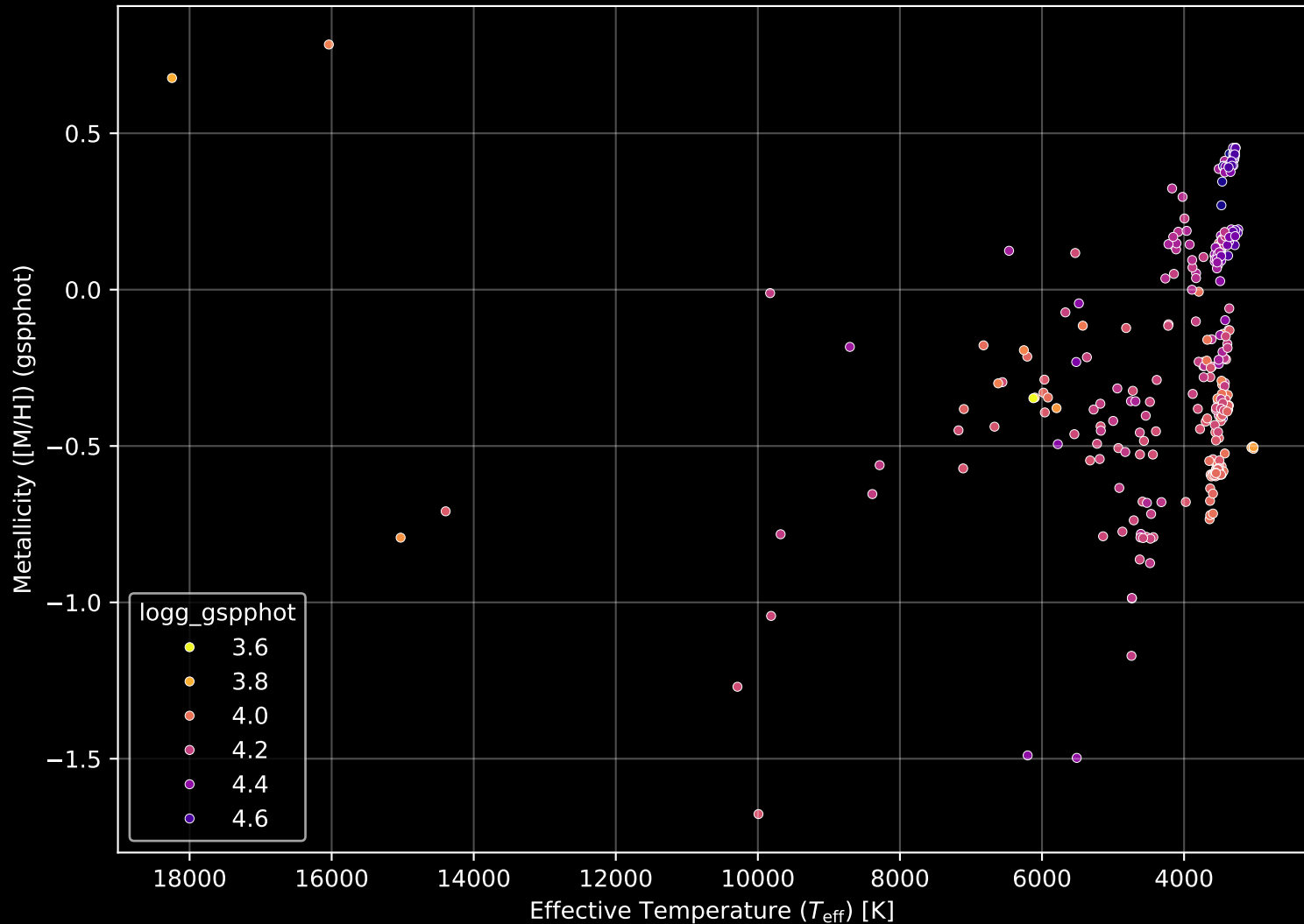
Gaia Cluster: [Pozzo_1] Stellar Population Parameters (n= 338)
