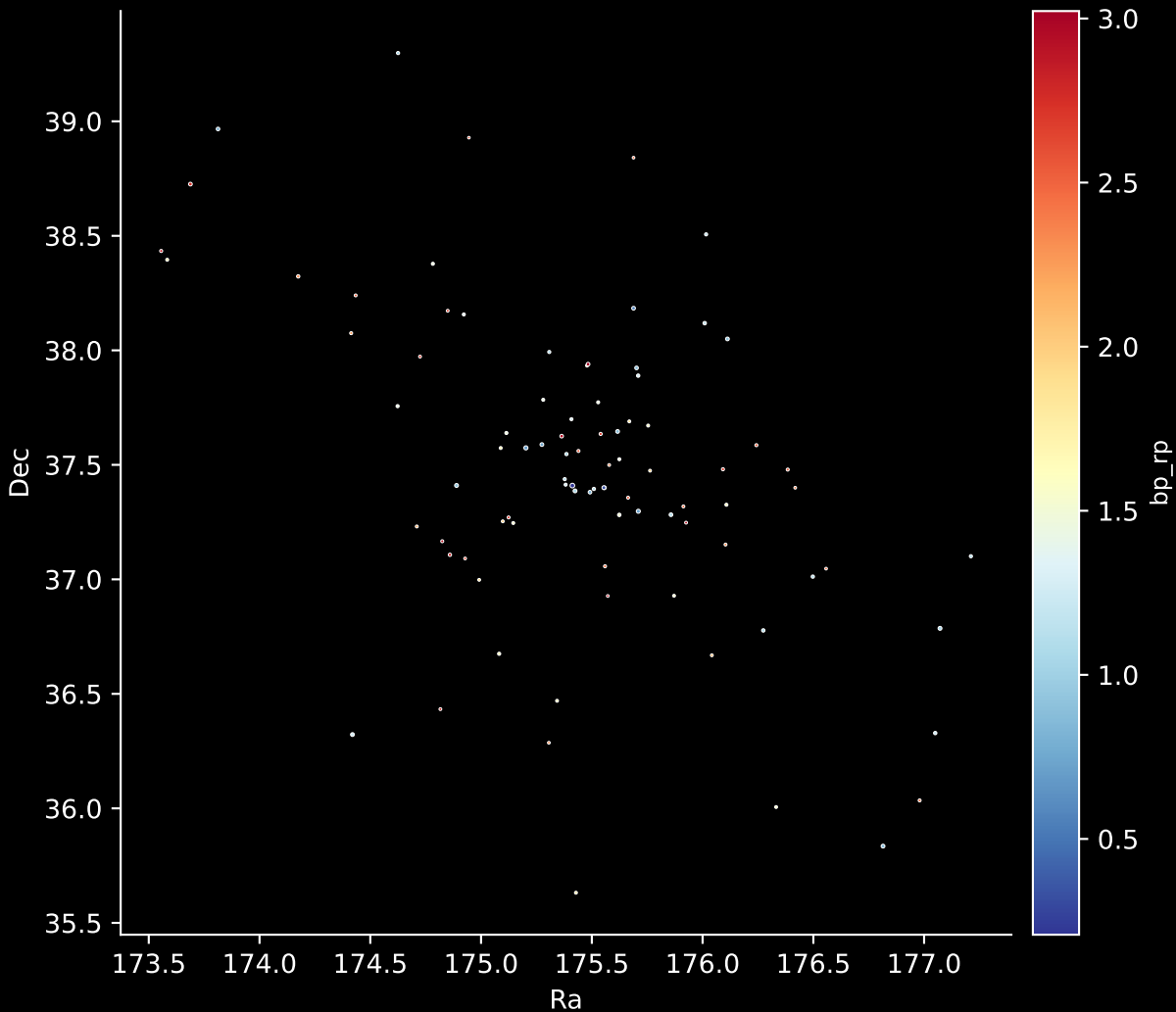
Gaia Cluster: [RSG_1] Stars: 89
