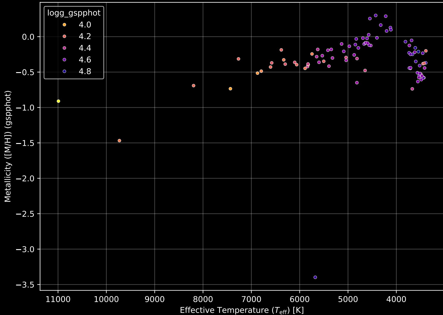
Gaia Cluster: [RSG_1] Stellar Population Parameters (n= 89)
