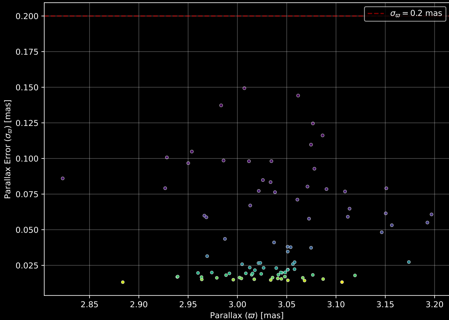
Gaia Cluster: [RSG_1] Parallax Quality (n= 89)
