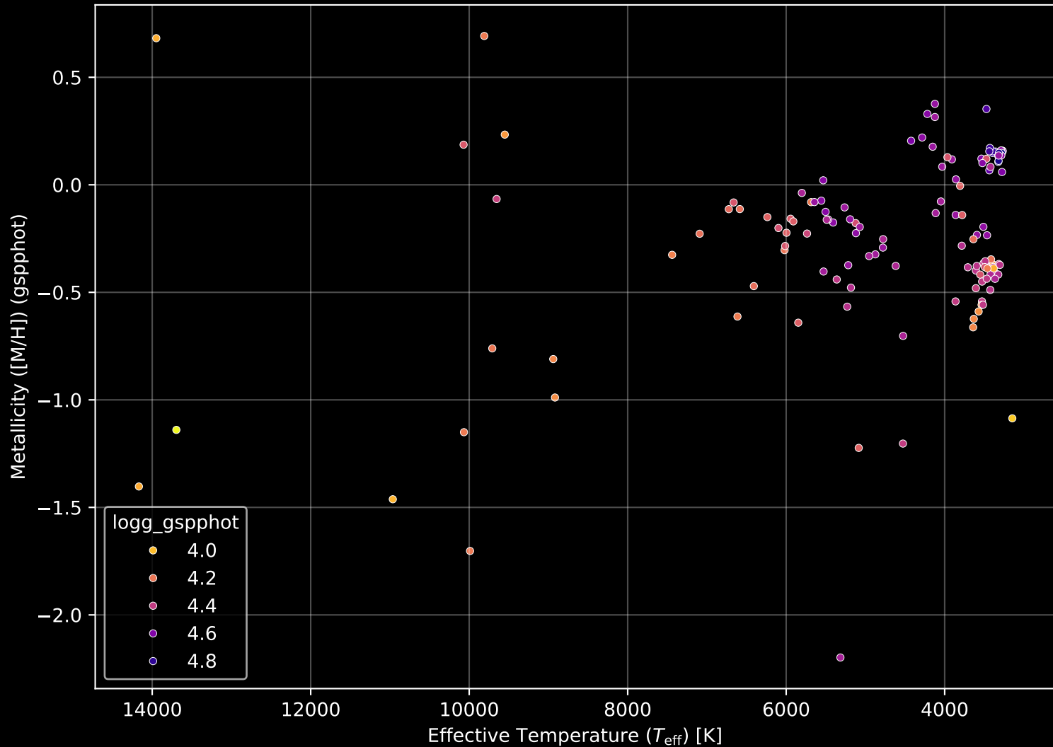
Gaia Cluster: [RSG_5] Stellar Population Parameters (n= 139)
