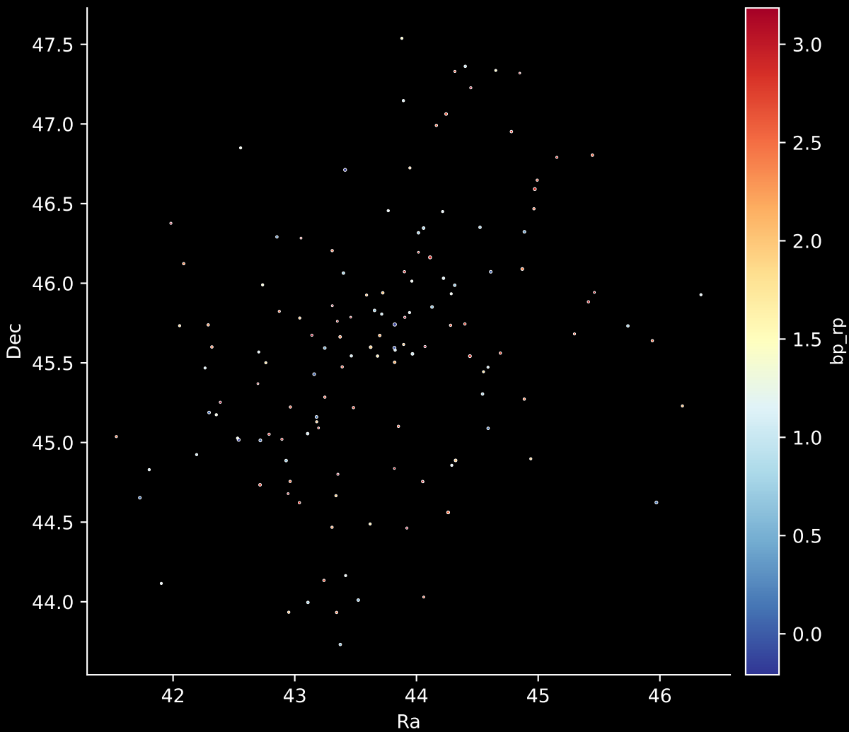
Gaia Cluster: [RSG_5] Stars: 139
