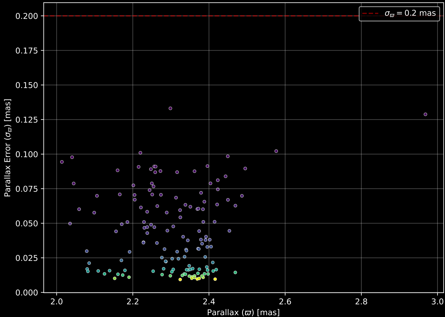
Gaia Cluster: [RSG_7] Parallax Quality (n= 143)
