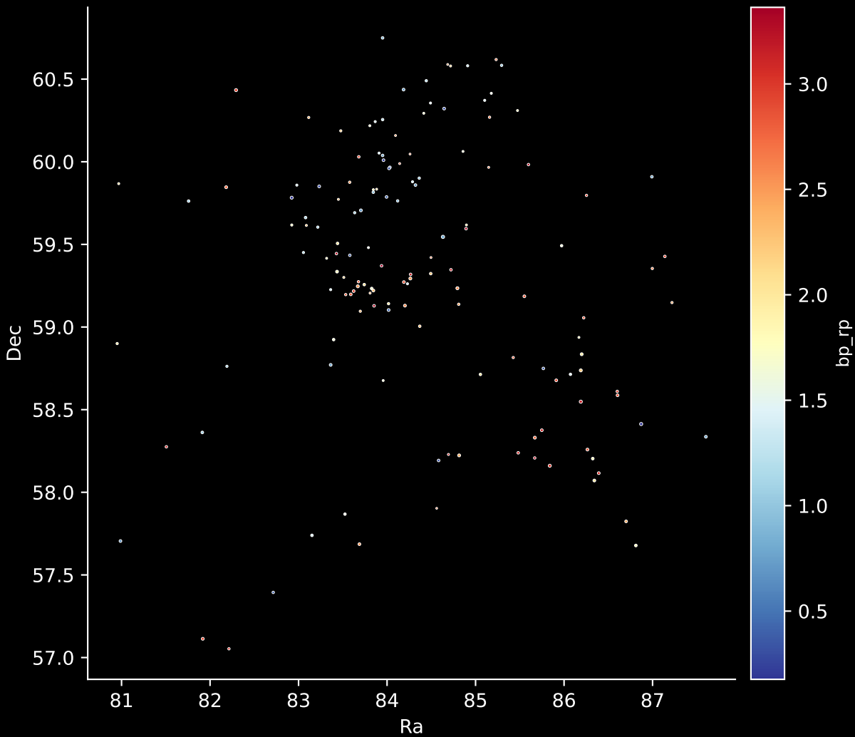
Gaia Cluster: [RSG_7] Stars: 143
