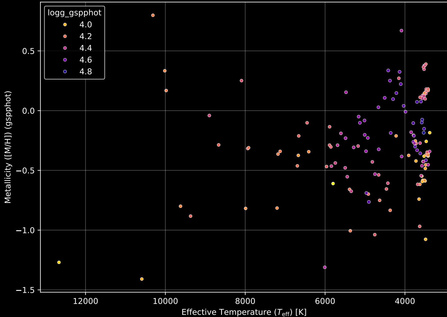
Gaia Cluster: [RSG_7] Stellar Population Parameters (n= 143)
