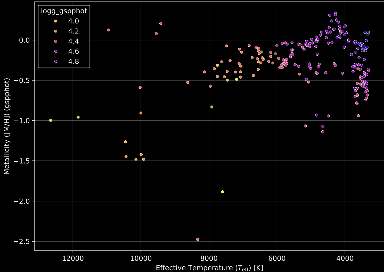
Gaia Cluster: [Roslund_6] Stellar Population Parameters (n= 229)
