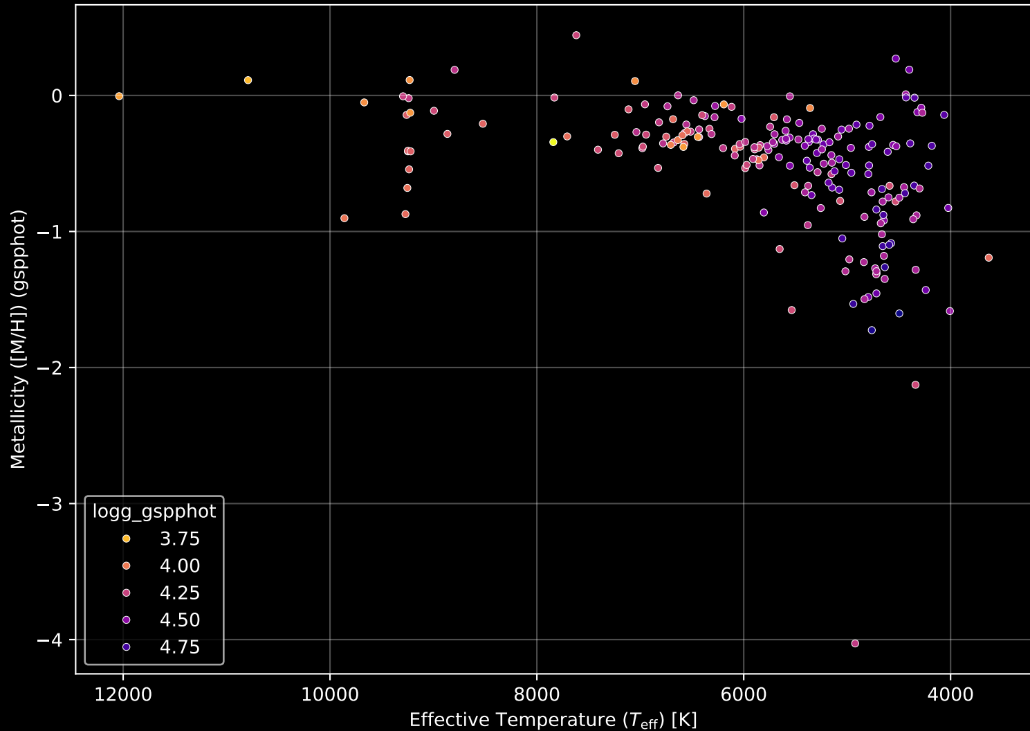
Gaia Cluster: [Roslund_7] Stellar Population Parameters (n= 208)
