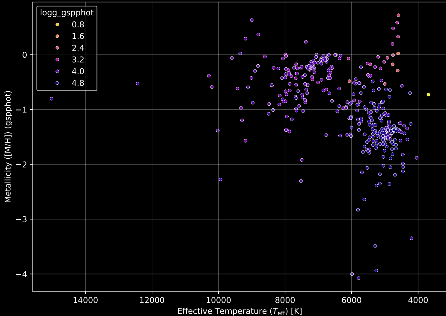
Gaia Cluster: [Ruprecht_105] Stellar Population Parameters (n= 385)
