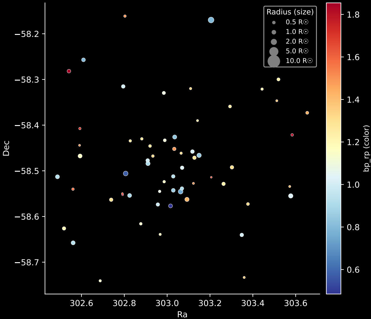
Gaia Cluster: [Ruprecht_108] Stars: 61
