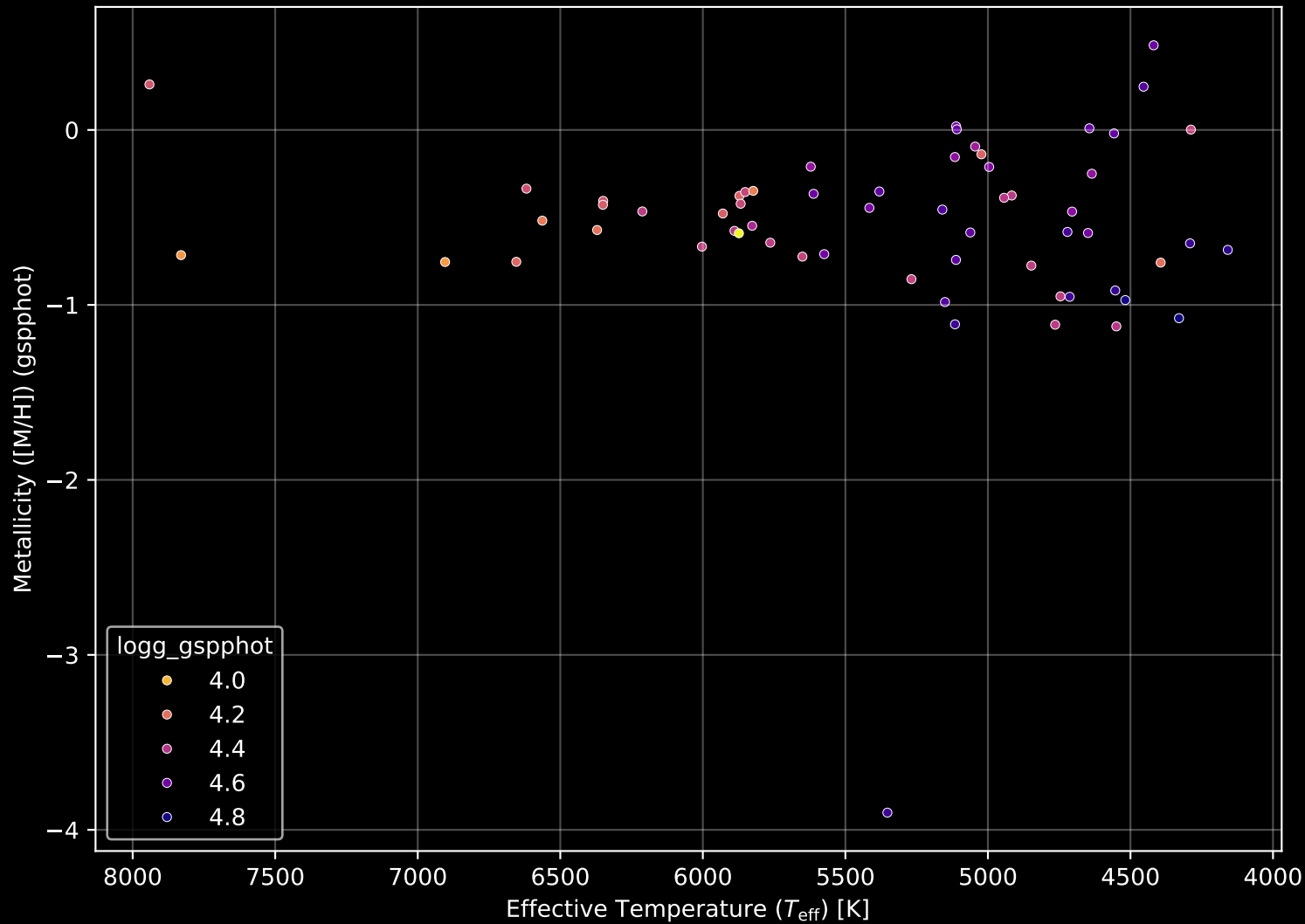
Gaia Cluster: [Ruprecht_108] Stellar Population Parameters (n= 61)
