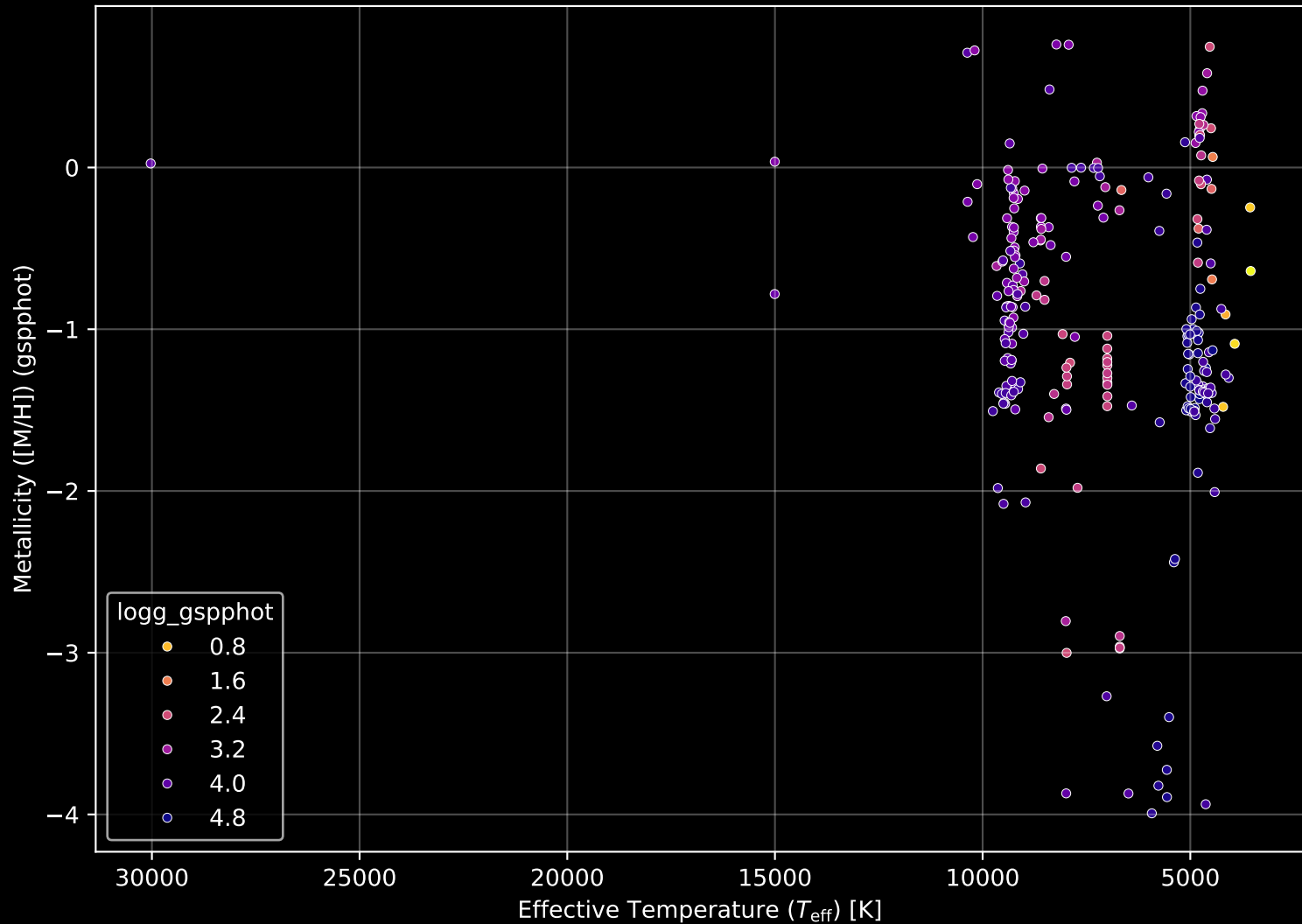
Gaia Cluster: [Ruprecht_126] Stellar Population Parameters (n= 270)
