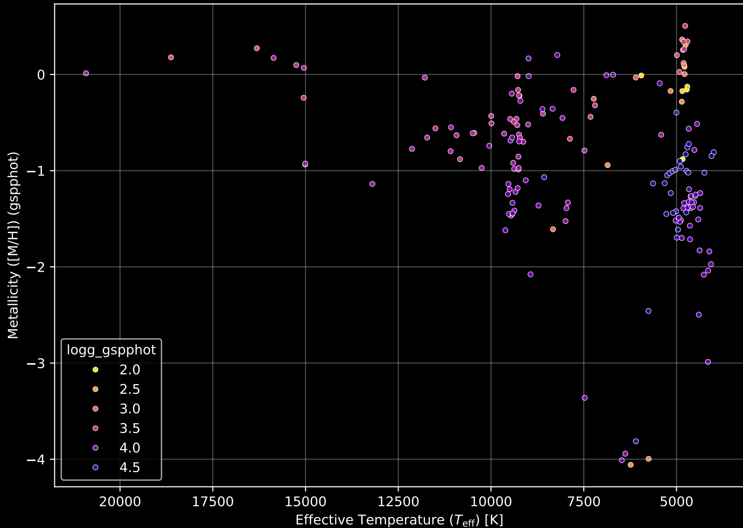
Gaia Cluster: [Ruprecht_127] Stellar Population Parameters (n= 173)
