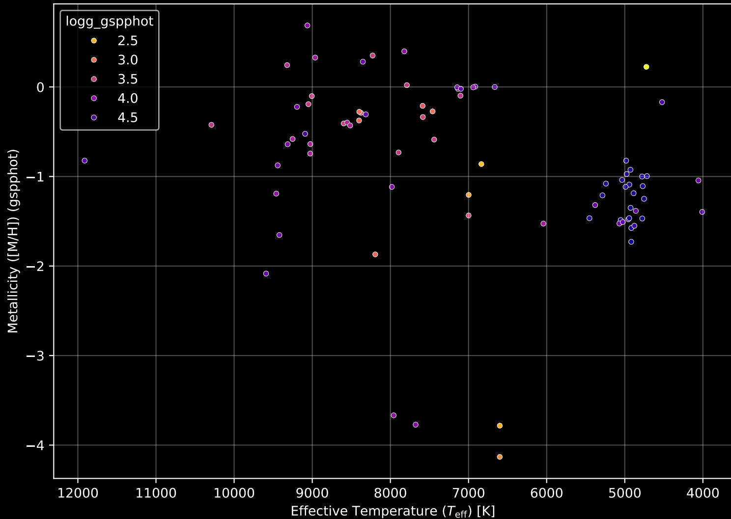
Gaia Cluster: [Ruprecht_130] Stellar Population Parameters (n= 80)
