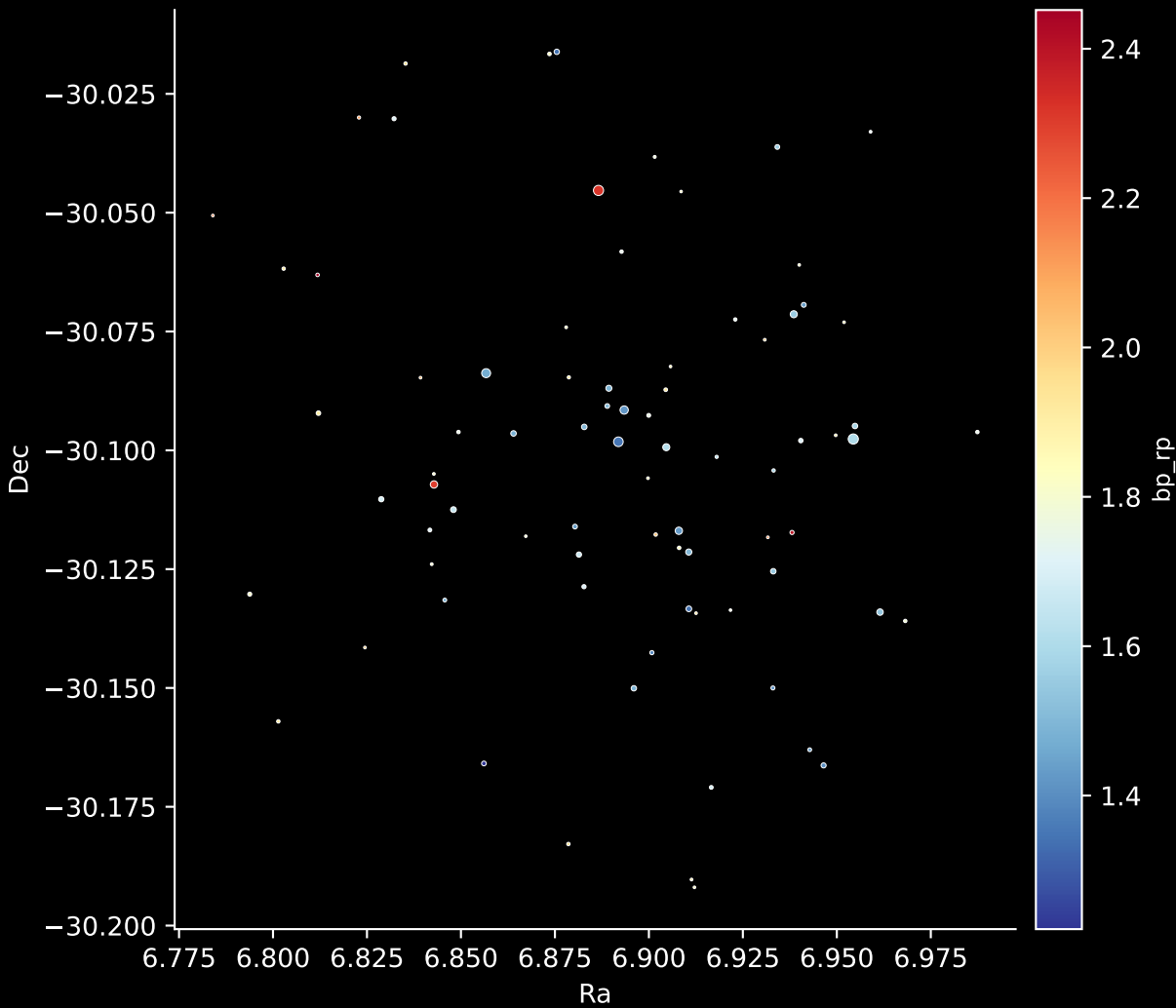
Gaia Cluster: [Ruprecht_130] Stars: 80
