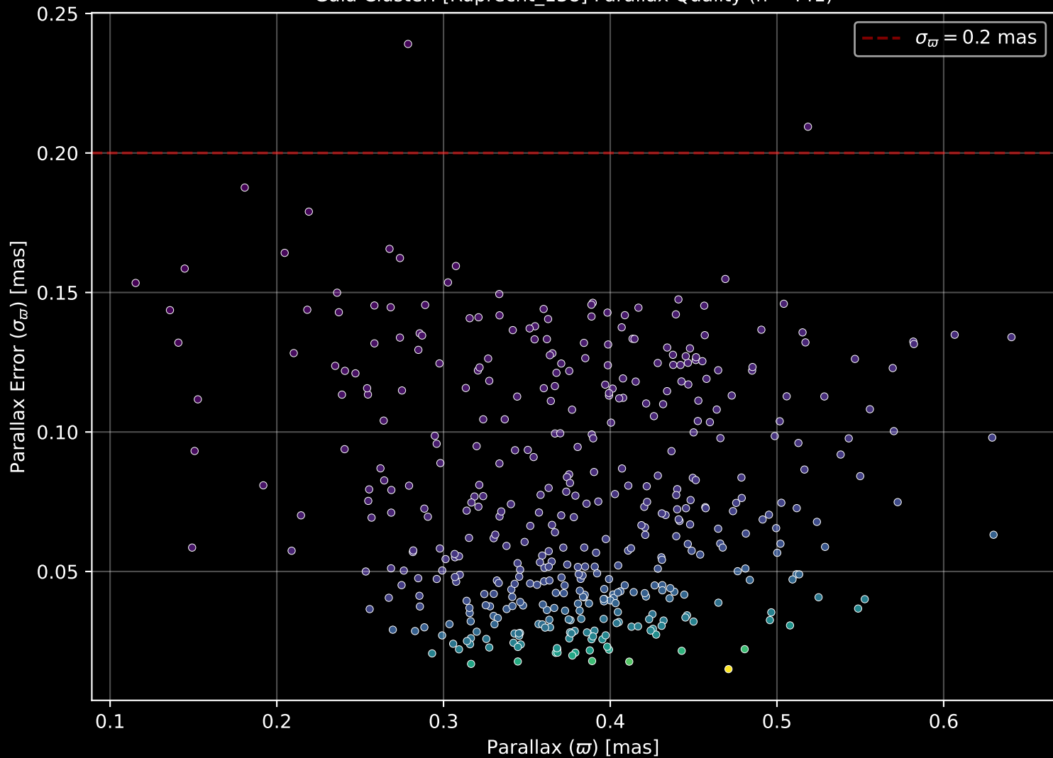
Gaia Cluster: [Ruprecht_138] Parallax Quality (n= 441)
