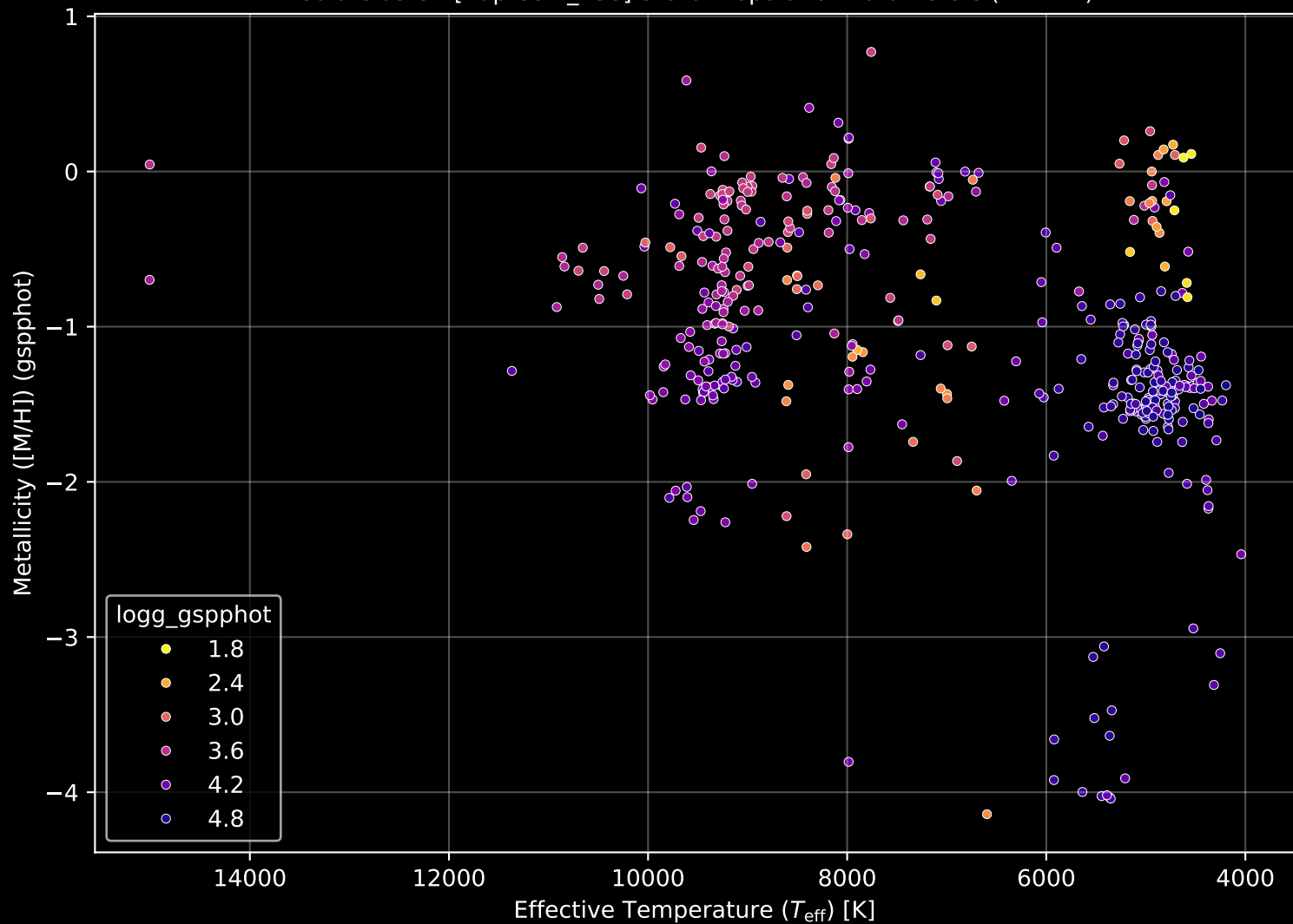
Gaia Cluster: [Ruprecht_138] Stellar Population Parameters (n= 441)
