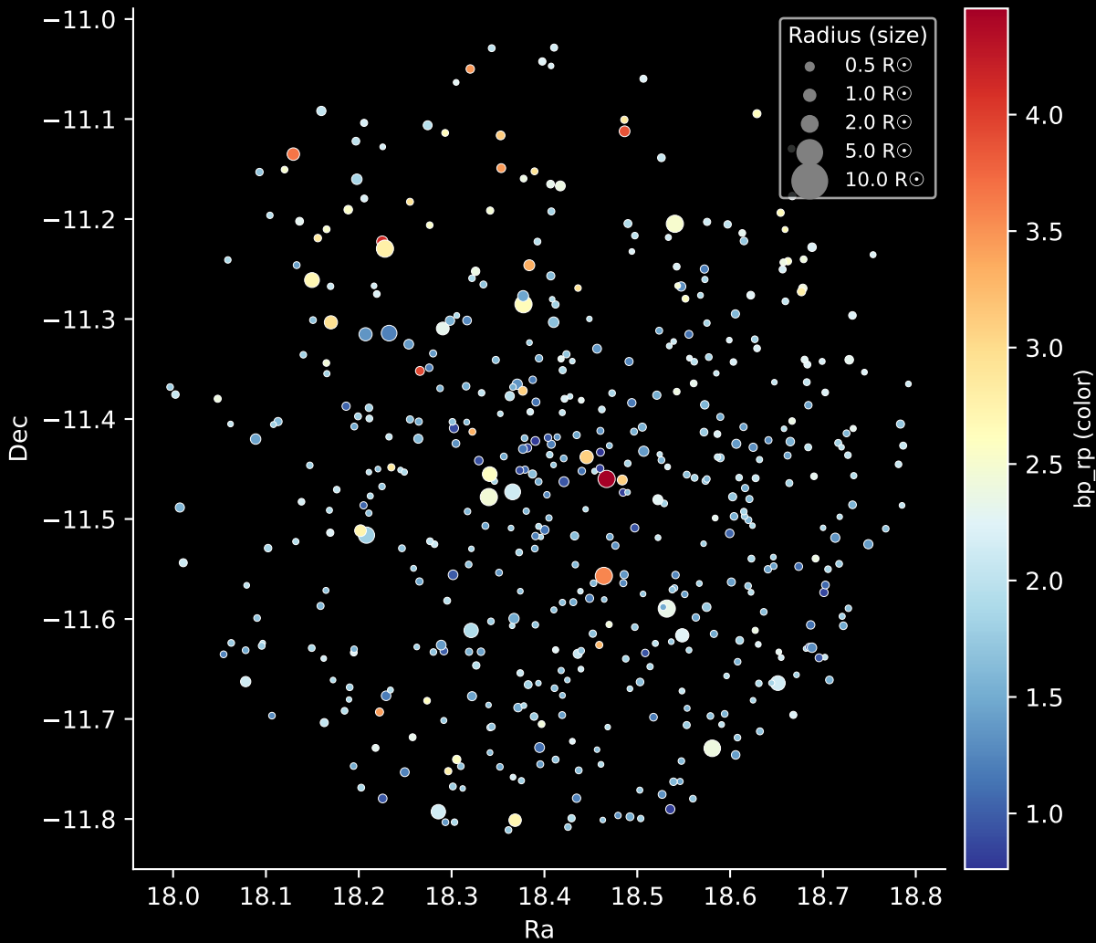
Gaia Cluster: [Ruprecht_144] Stars: 503
