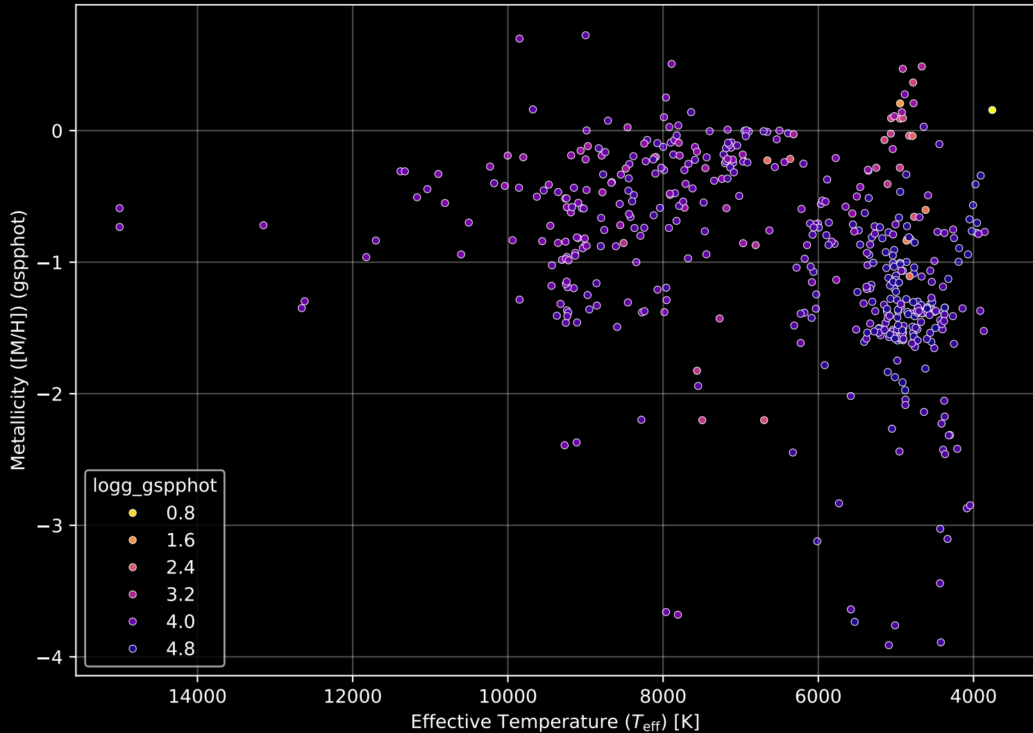
Gaia Cluster: [Ruprecht_144] Stellar Population Parameters (n= 503)
