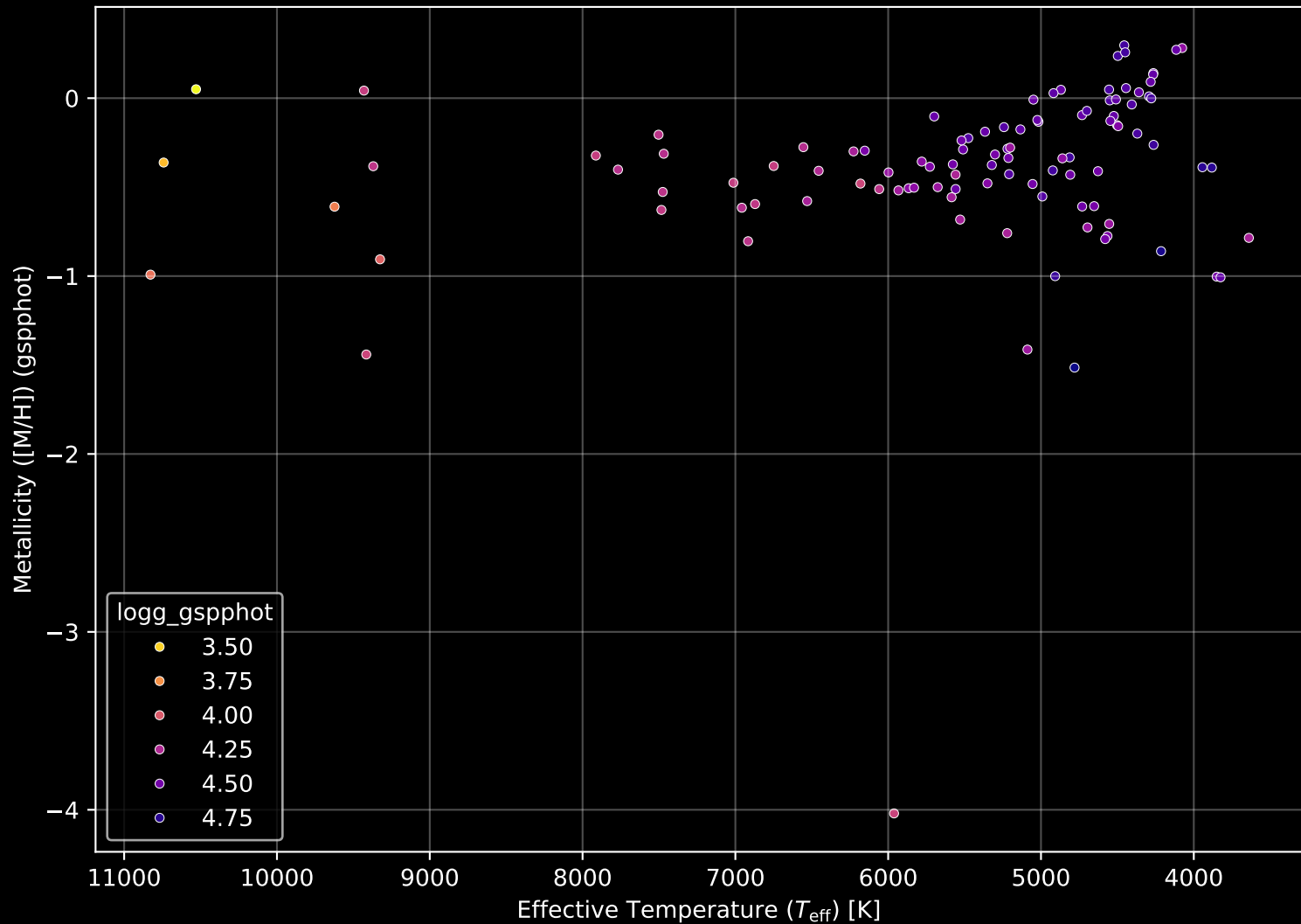
Gaia Cluster: [Ruprecht_161] Stellar Population Parameters (n= 105)
