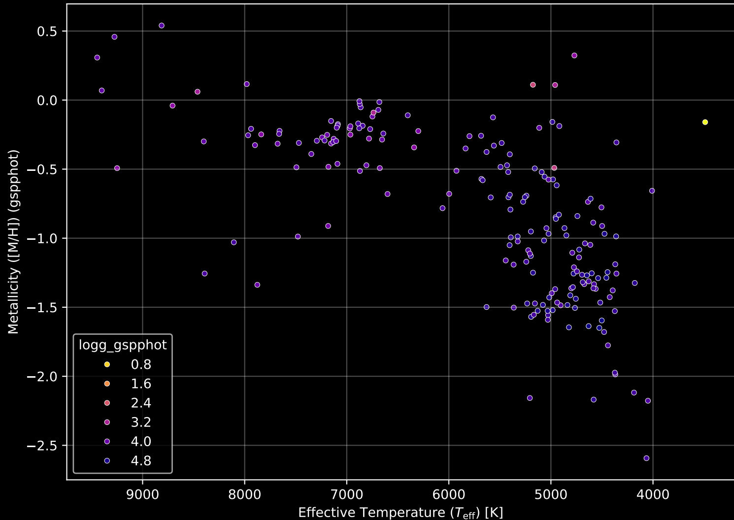
Gaia Cluster: [Ruprecht_167] Stellar Population Parameters (n= 193)
