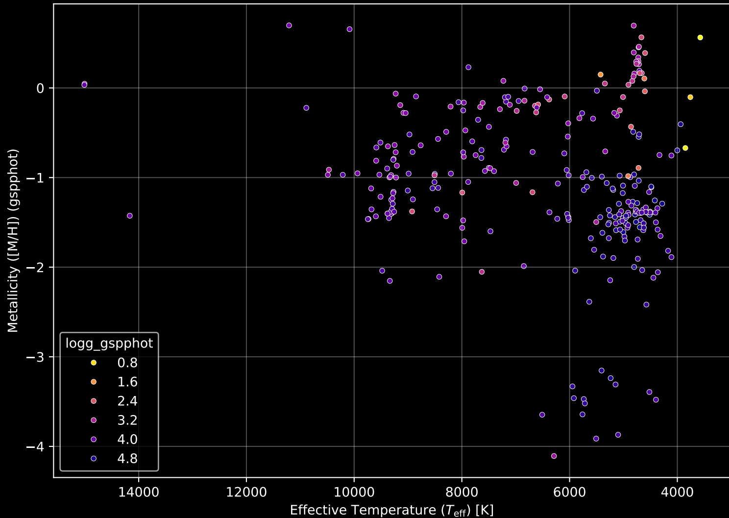
Gaia Cluster: [Ruprecht_170] Stellar Population Parameters (n= 288)
