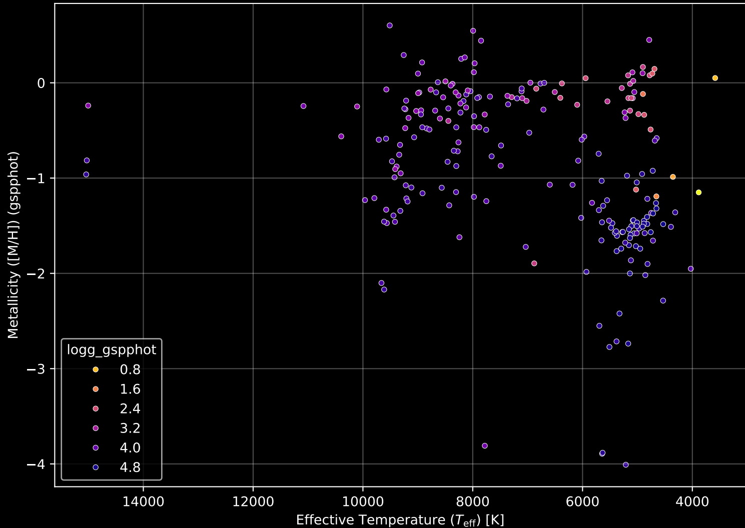
Gaia Cluster: [Ruprecht_172] Stellar Population Parameters (n= 224)
