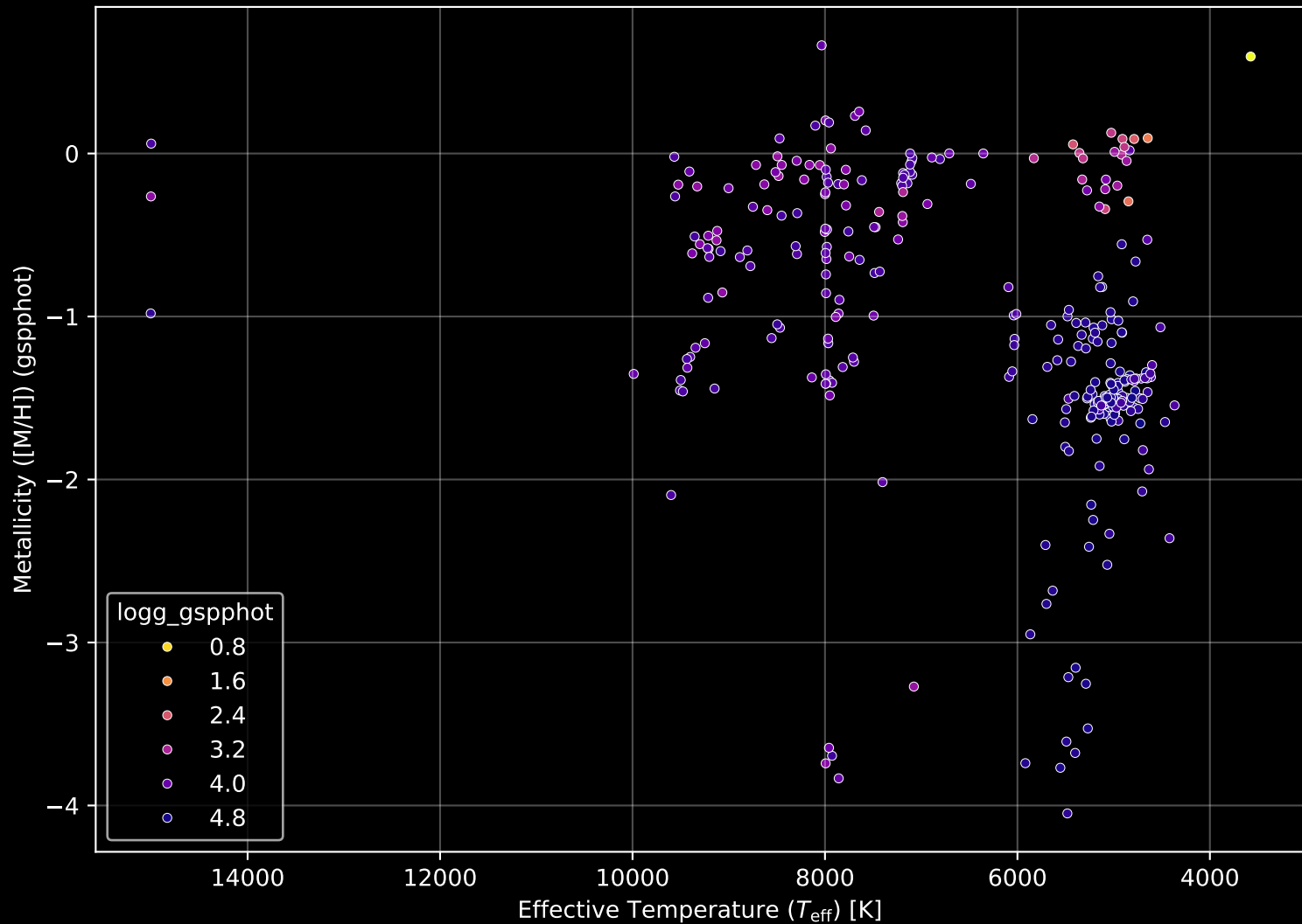
Gaia Cluster: [Ruprecht_174] Stellar Population Parameters (n= 311)
