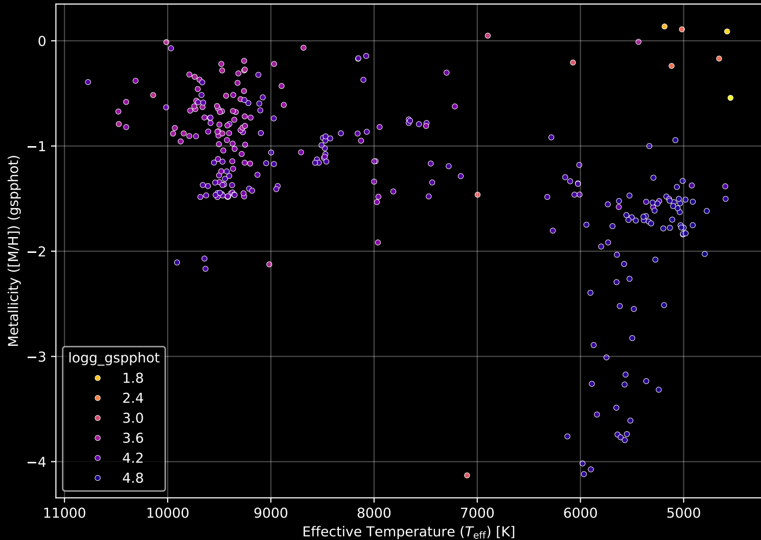
Gaia Cluster: [Ruprecht_18] Stellar Population Parameters (n= 279)
