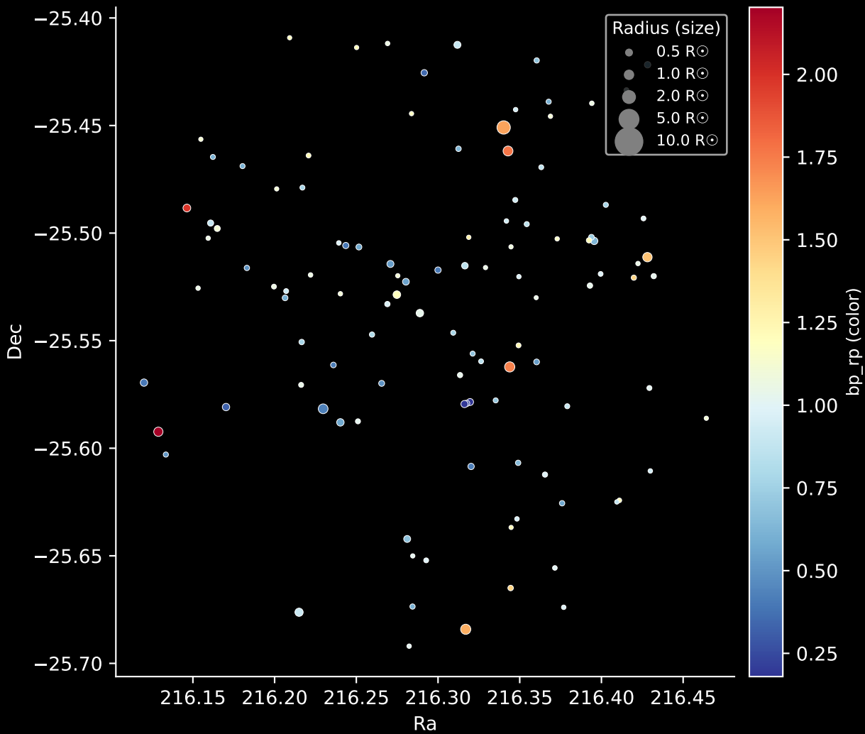
Gaia Cluster: [Ruprecht_32] Stars: 110
