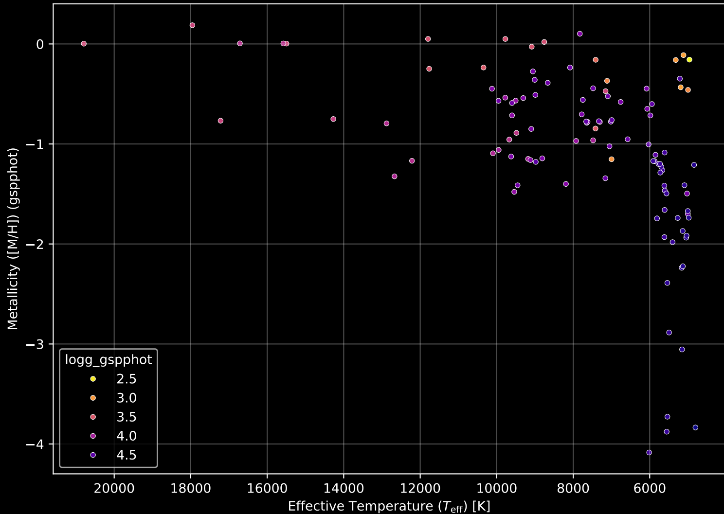
Gaia Cluster: [Ruprecht_32] Stellar Population Parameters (n= 110)
