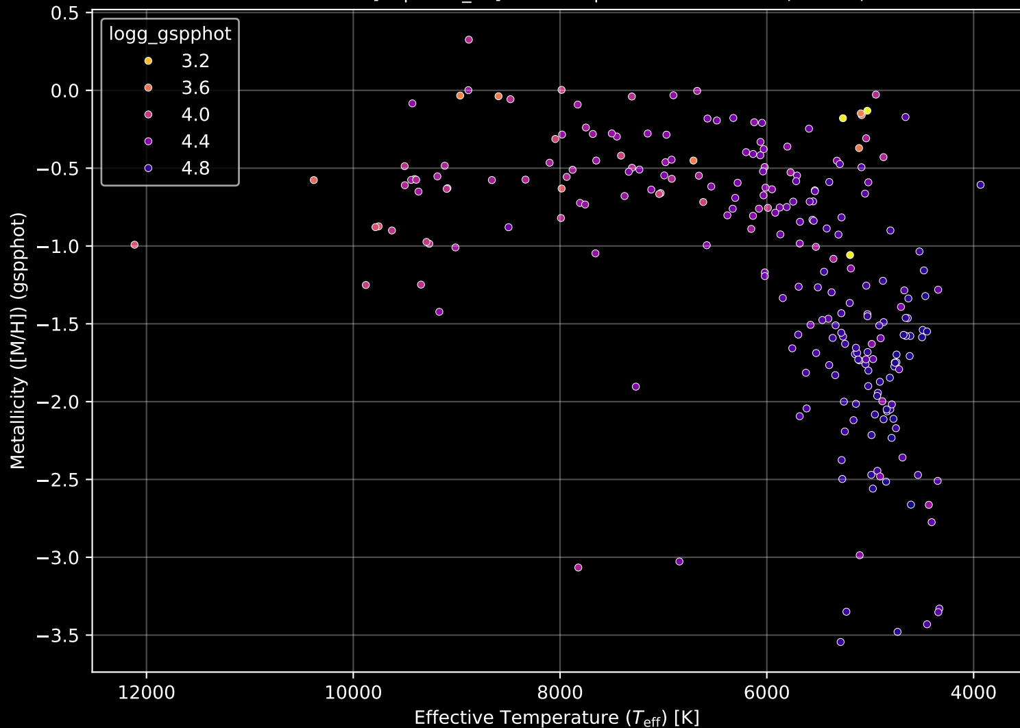
Gaia Cluster: [Ruprecht_33] Stellar Population Parameters (n= 242)
