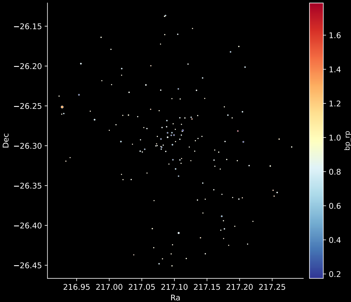
Gaia Cluster: [Ruprecht_36] Stars: 152
