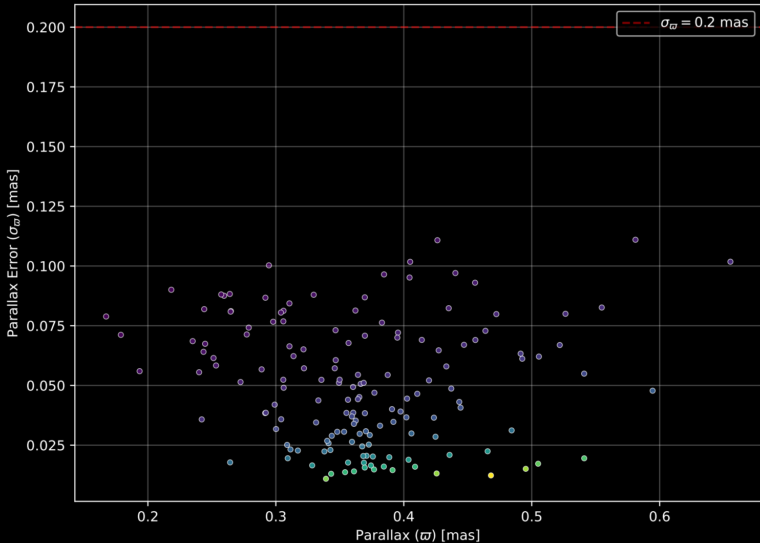
Gaia Cluster: [Ruprecht_36] Parallax Quality (n= 152)
