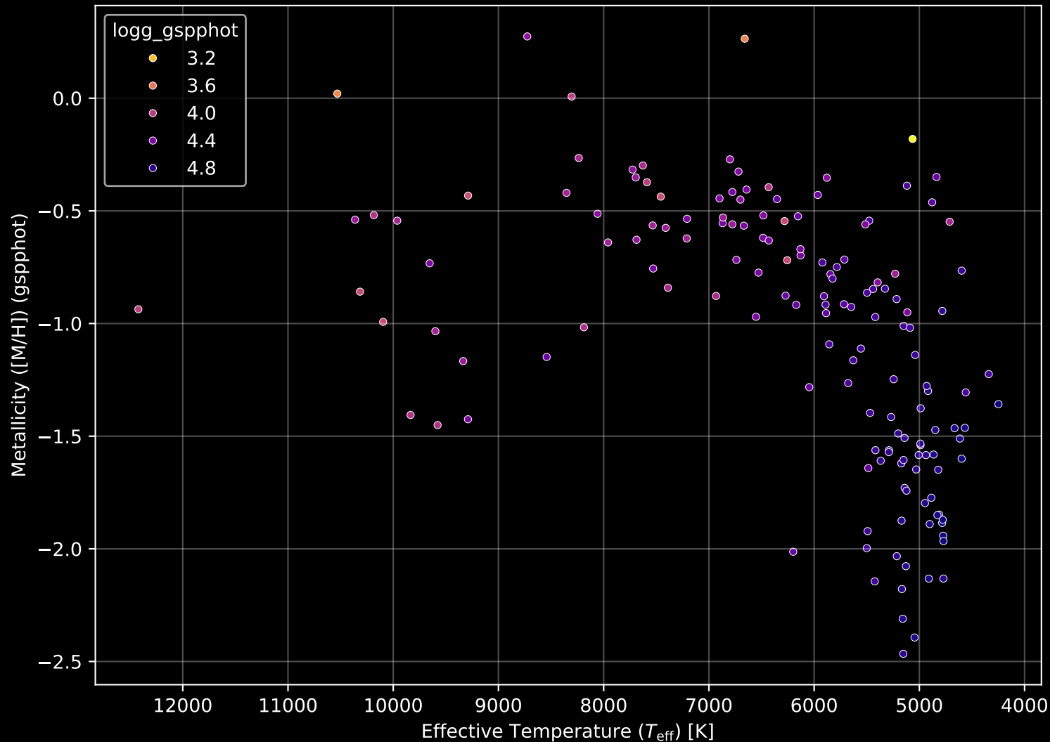
Gaia Cluster: [Ruprecht_36] Stellar Population Parameters (n= 152)
