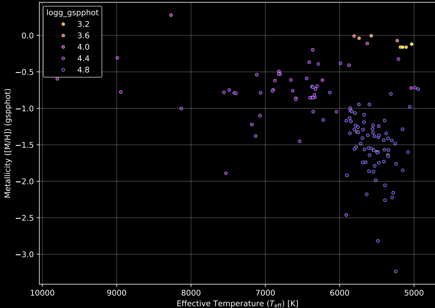
Gaia Cluster: [Ruprecht_37] Stellar Population Parameters (n= 130)
