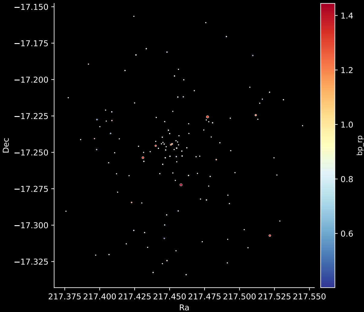
Gaia Cluster: [Ruprecht_37] Stars: 130
