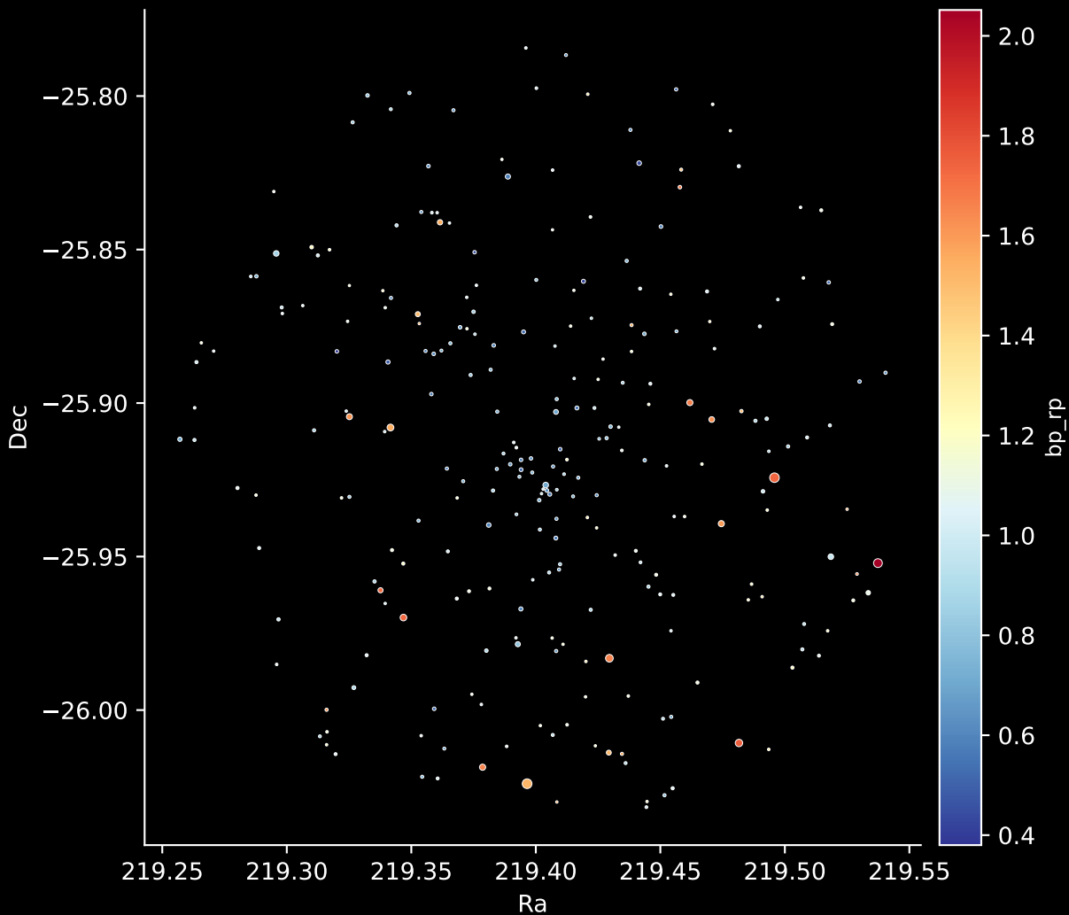
Gaia Cluster: [Ruprecht_42] Stars: 260
