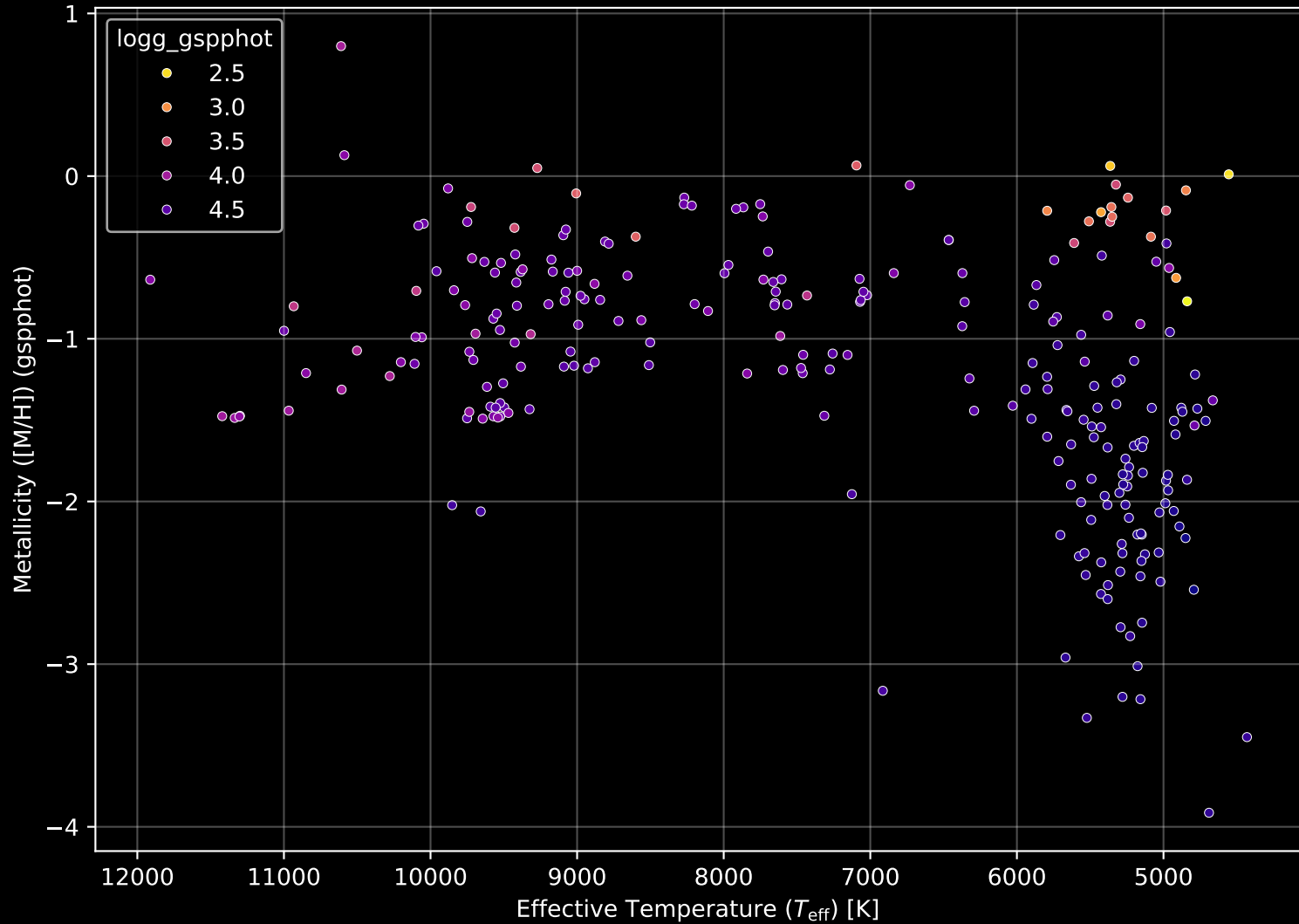
Gaia Cluster: [Ruprecht_42] Stellar Population Parameters (n= 260)
