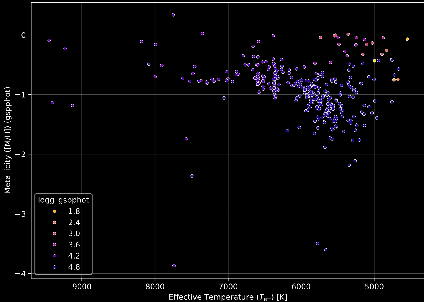
Gaia Cluster: [Ruprecht_45] Stellar Population Parameters (n= 322)
