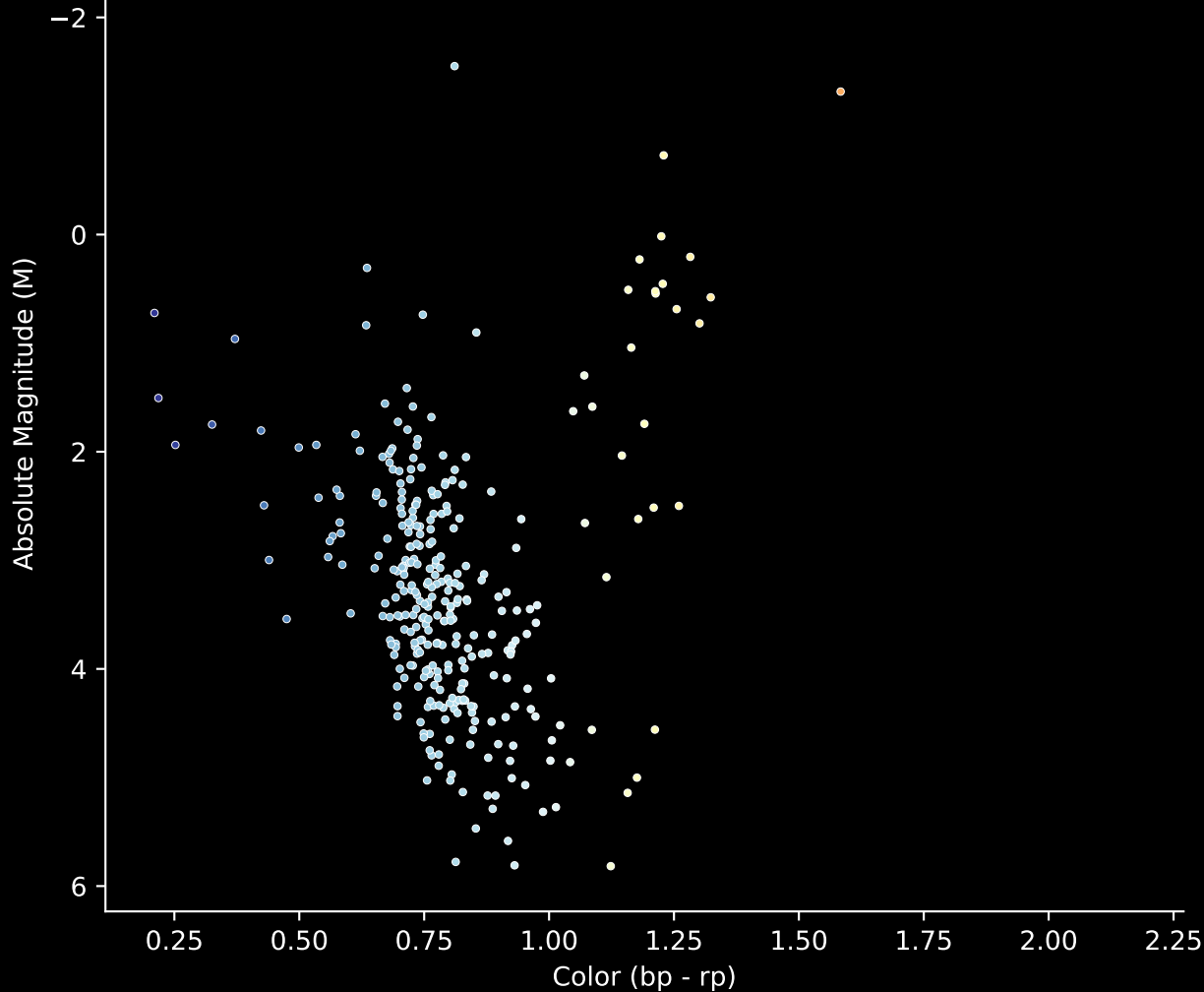
Gaia Cluster: [Ruprecht_45] Stars (n= 322) Hertzsprung-Russel Diagram
