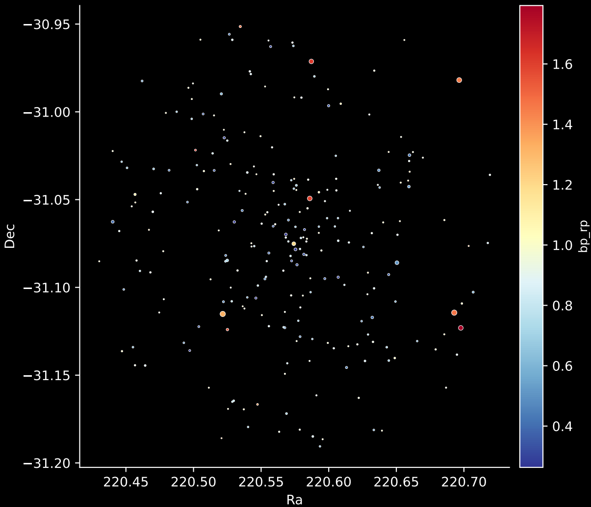
Gaia Cluster: [Ruprecht_47] Stars: 245
