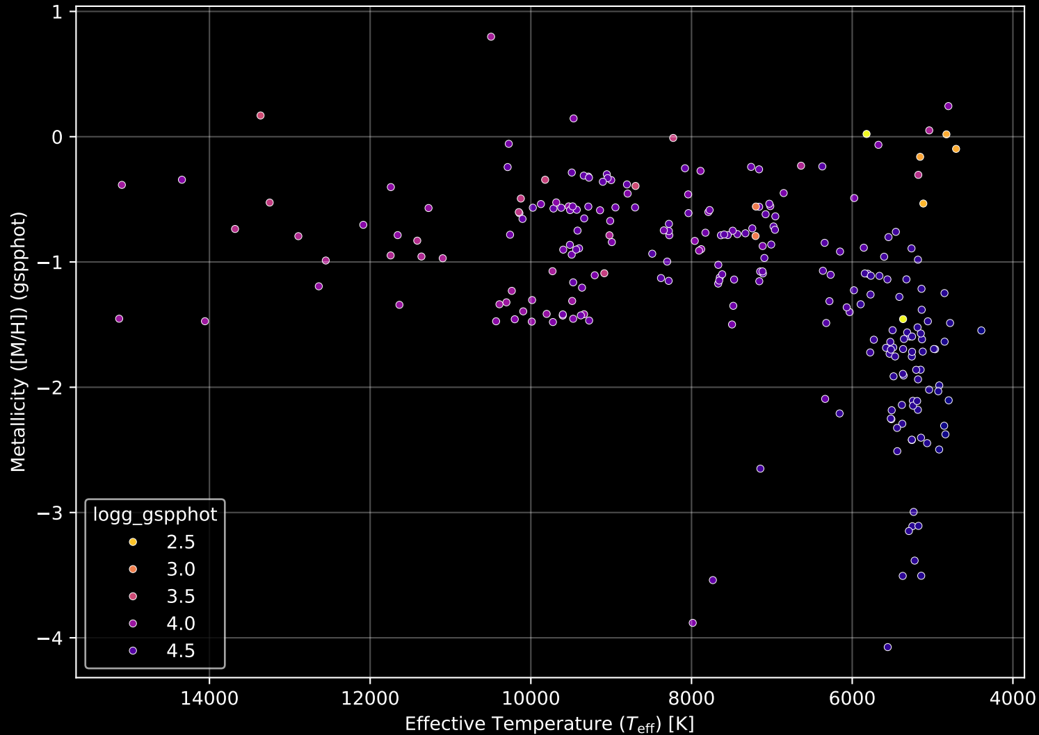
Gaia Cluster: [Ruprecht_47] Stellar Population Parameters (n= 245)
