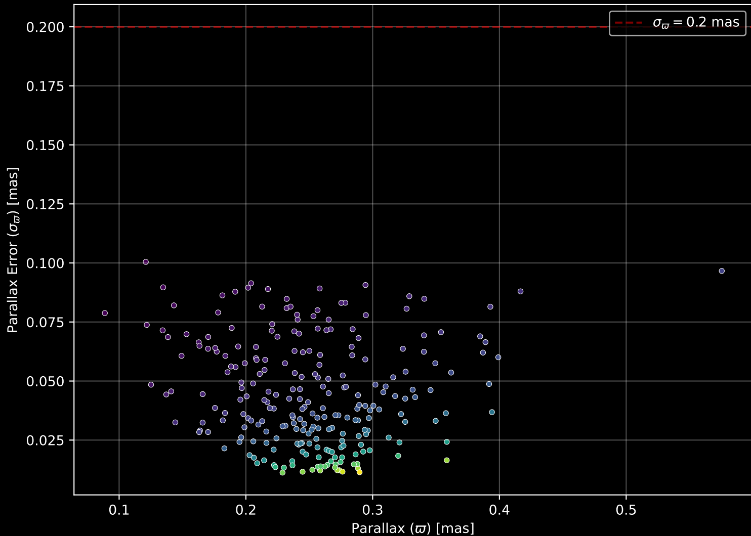
Gaia Cluster: [Ruprecht_47] Parallax Quality (n= 245)
