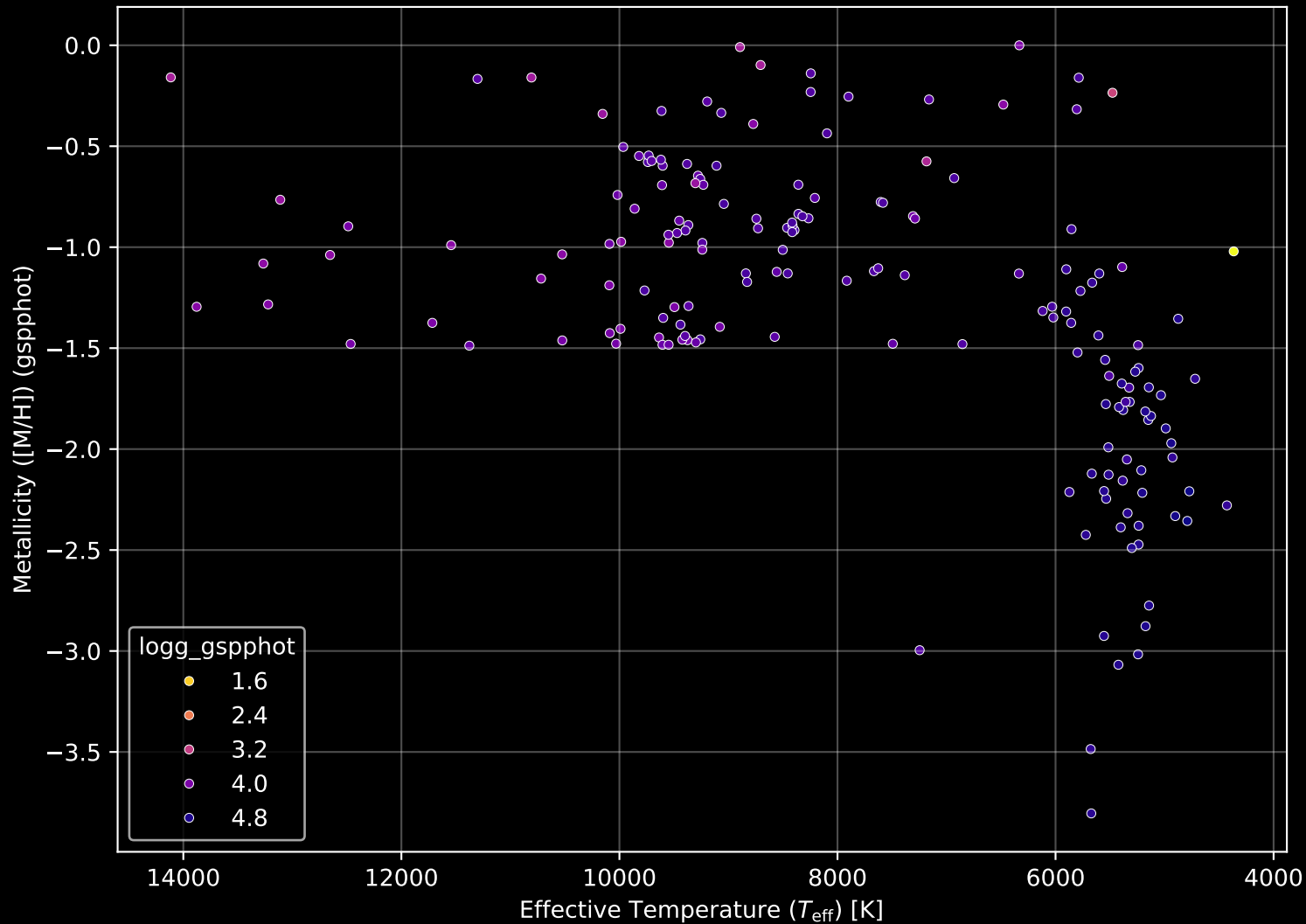
Gaia Cluster: [Ruprecht_48] Stellar Population Parameters (n= 174)
