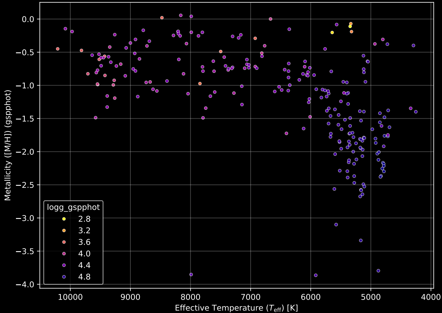
Gaia Cluster: [Ruprecht_58] Stellar Population Parameters (n= 234)
