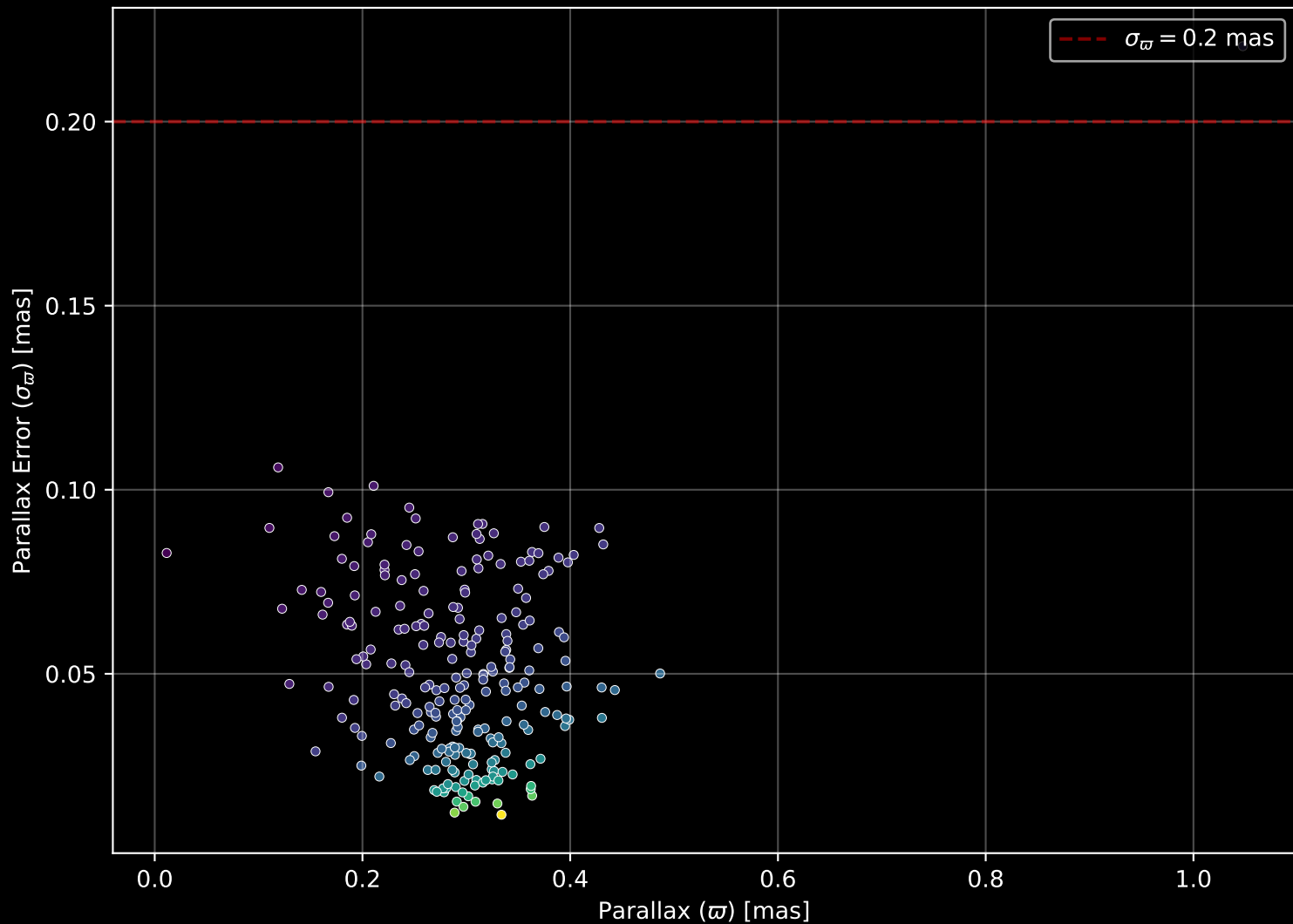
Gaia Cluster: [Ruprecht_58] Parallax Quality (n= 234)
