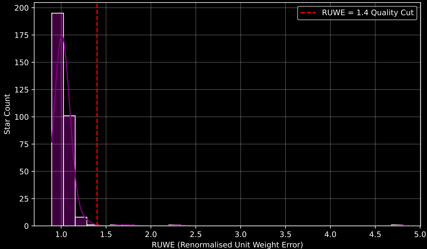
Gaia Cluster: [Ruprecht_60] RUWE Distribution (n= 309)
