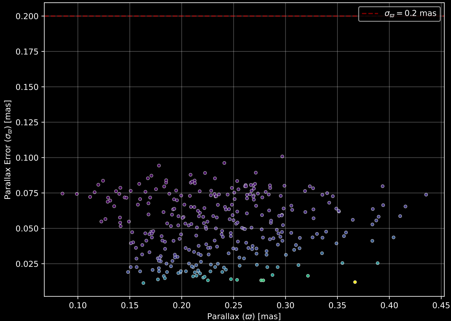
Gaia Cluster: [Ruprecht_60] Parallax Quality (n= 309)
