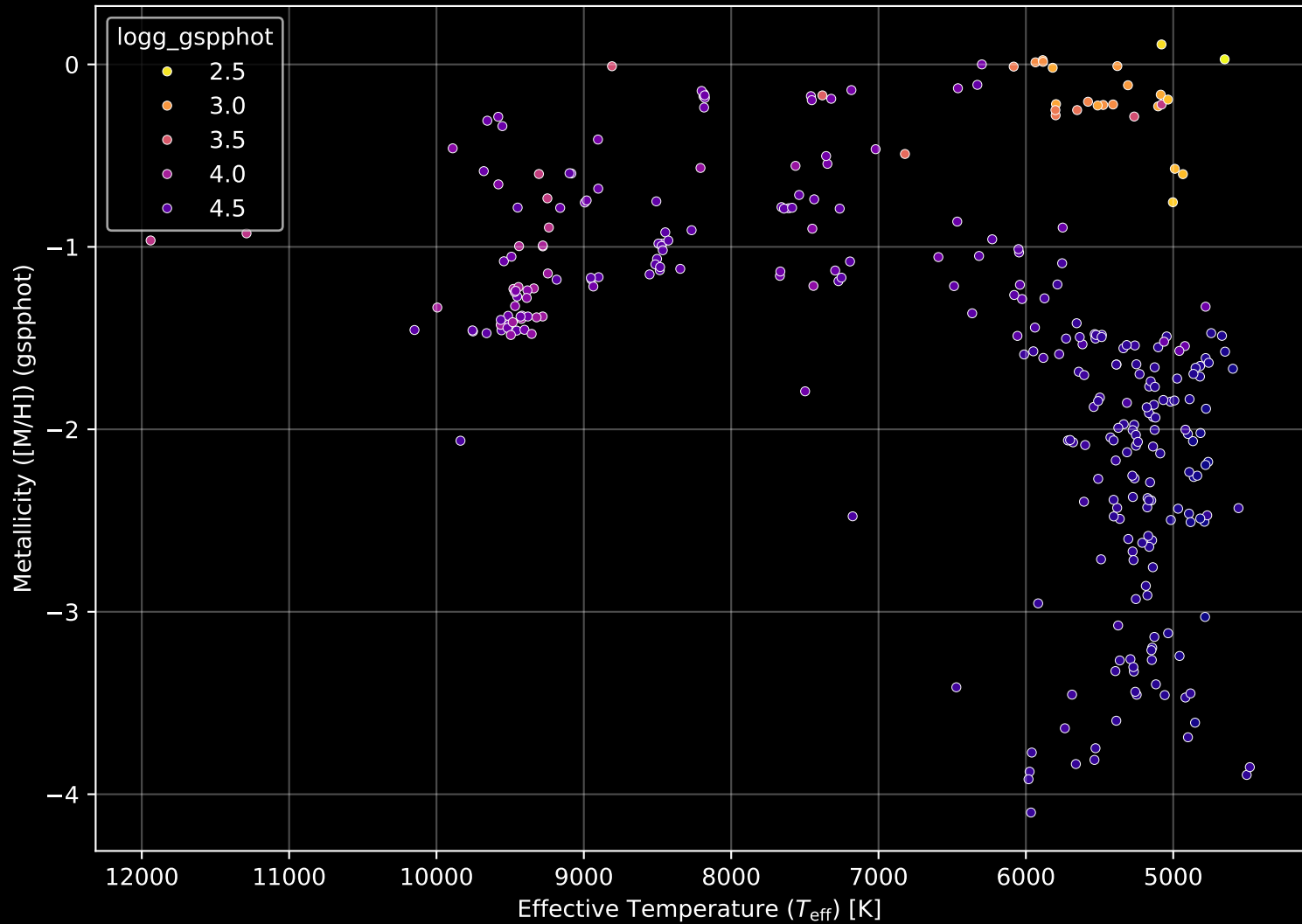
Gaia Cluster: [Ruprecht_60] Stellar Population Parameters (n= 309)
