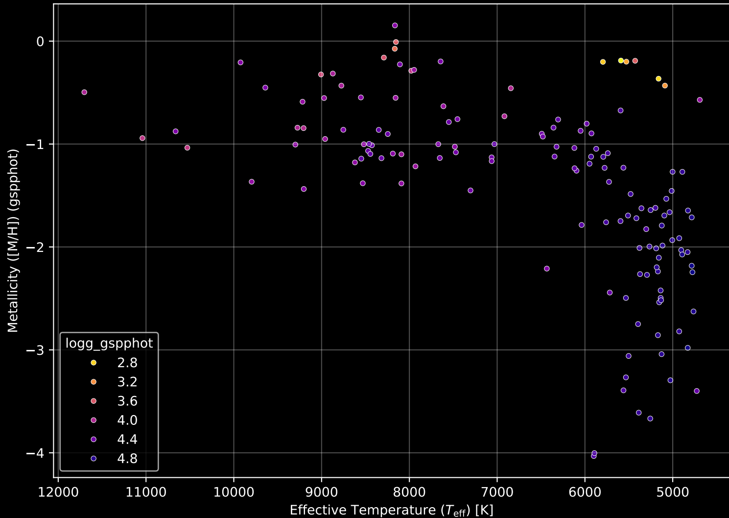
Gaia Cluster: [Ruprecht_61] Stellar Population Parameters (n= 141)
