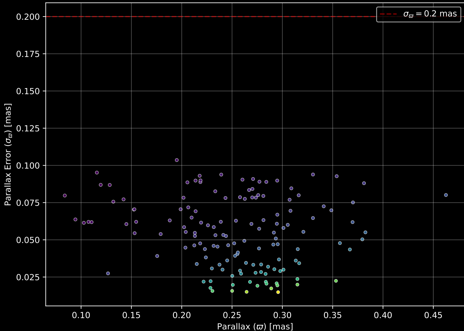
Gaia Cluster: [Ruprecht_61] Parallax Quality (n= 141)
