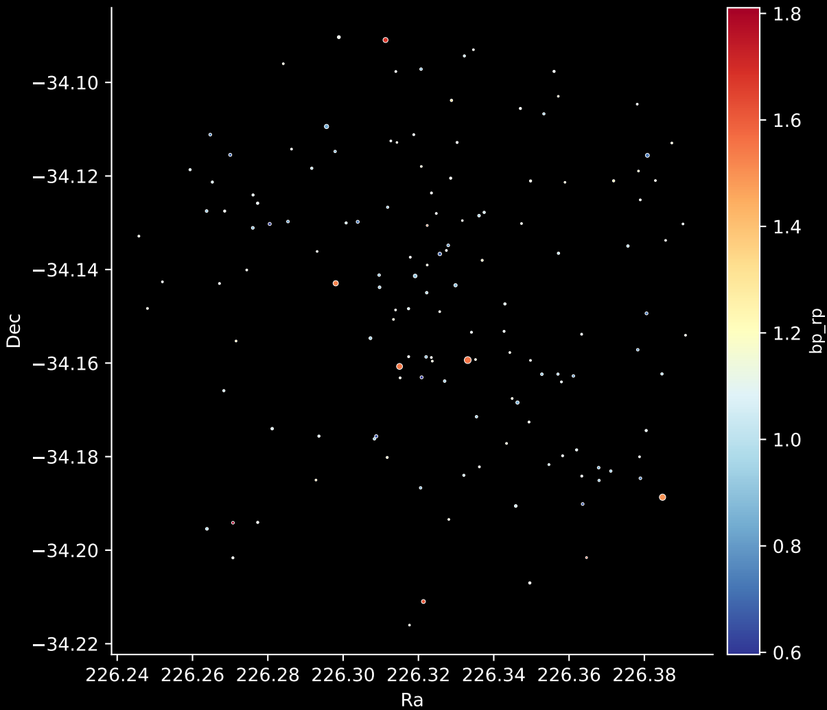
Gaia Cluster: [Ruprecht_61] Stars: 141
