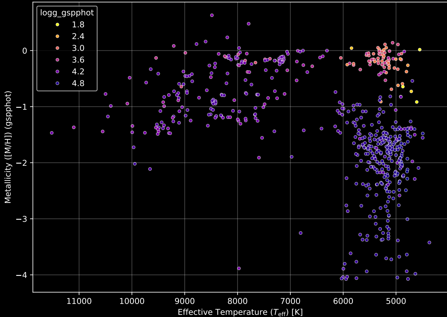
Gaia Cluster: [Ruprecht_66] Stellar Population Parameters (n= 577)
