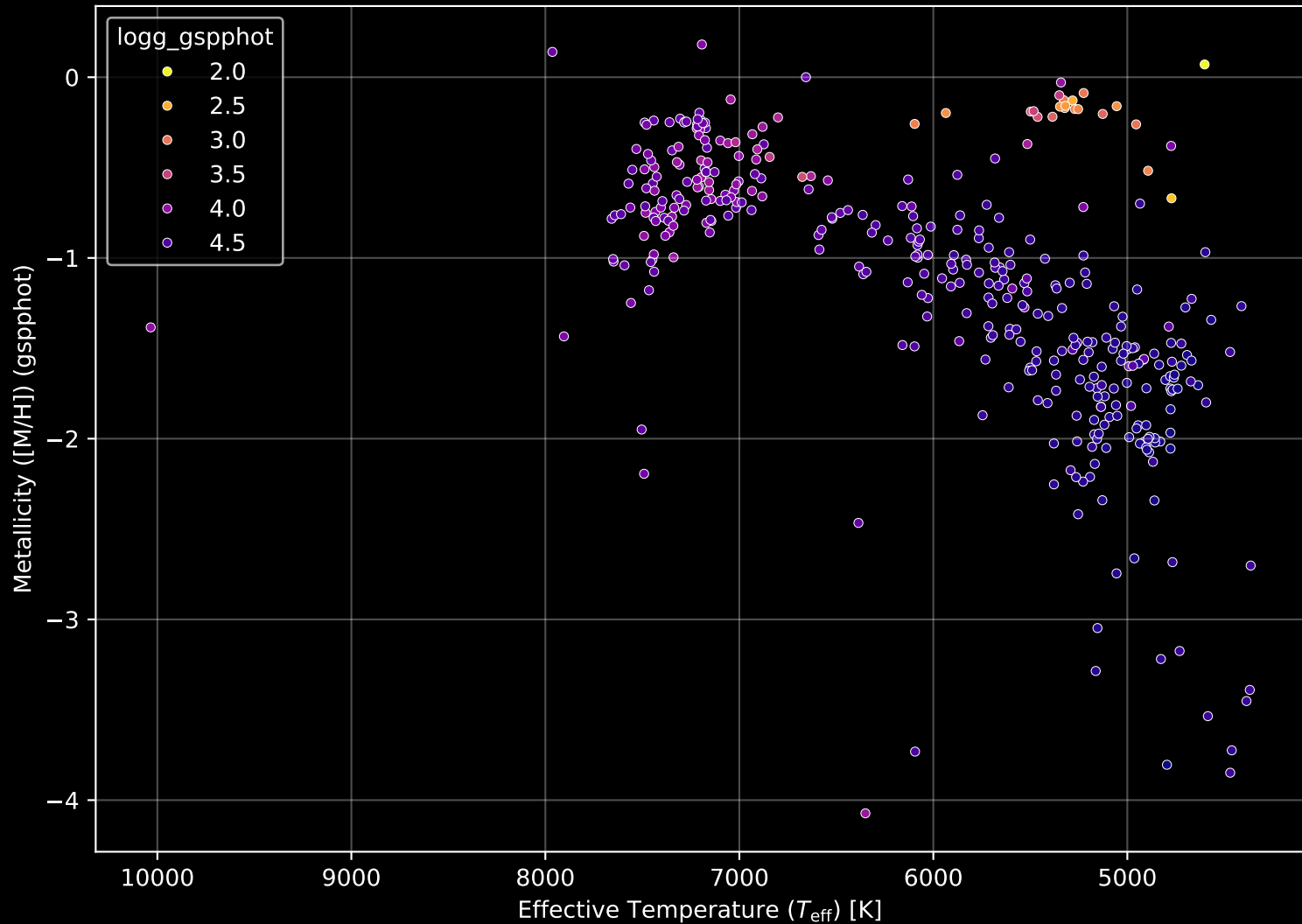
Gaia Cluster: [Ruprecht_68] Stellar Population Parameters (n= 382)
