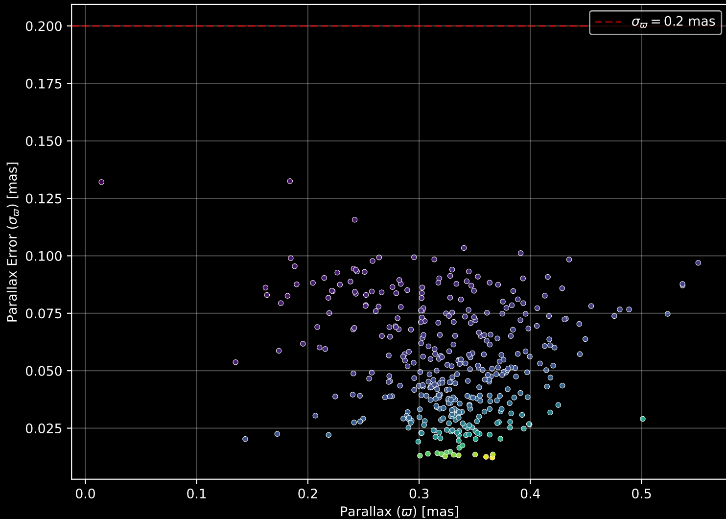
Gaia Cluster: [Ruprecht_68] Parallax Quality (n= 382)
